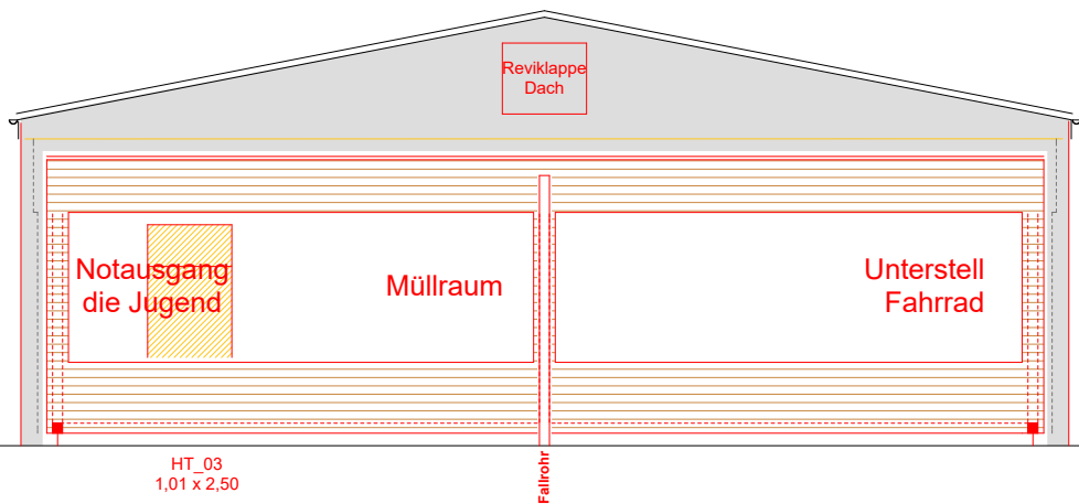
Ansicht West
