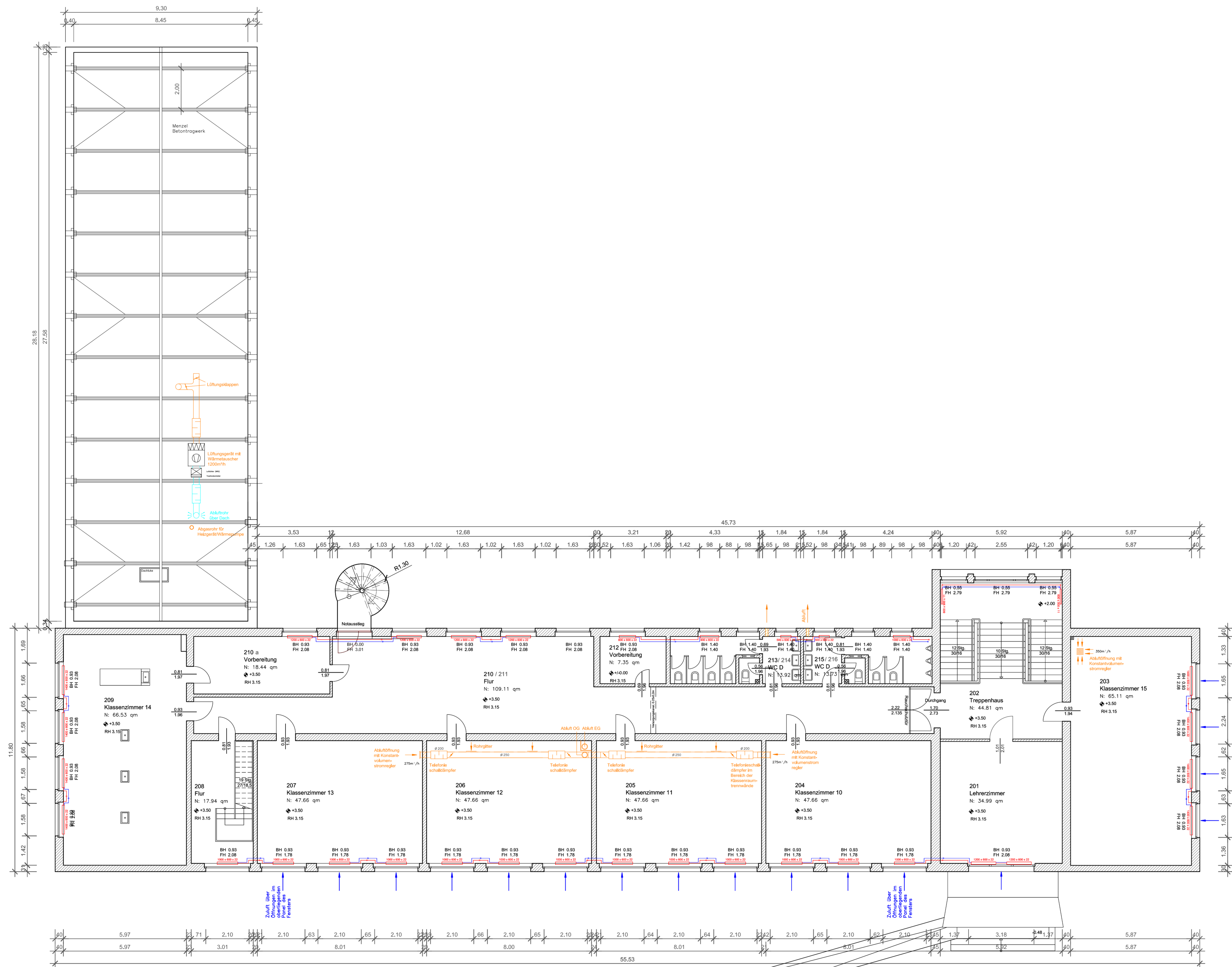
Grundriss OG 1:100
