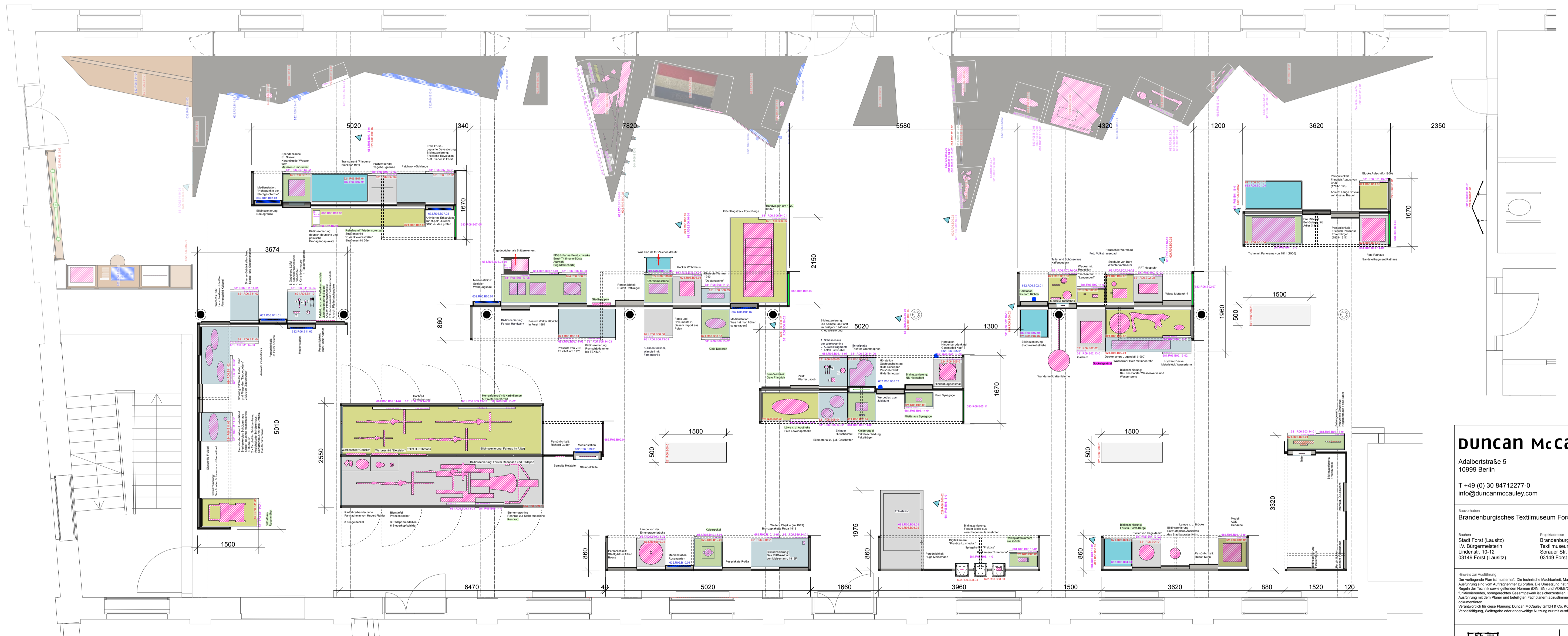
Grundriss Kapitel 6.1 & 6.3 M 1:50
