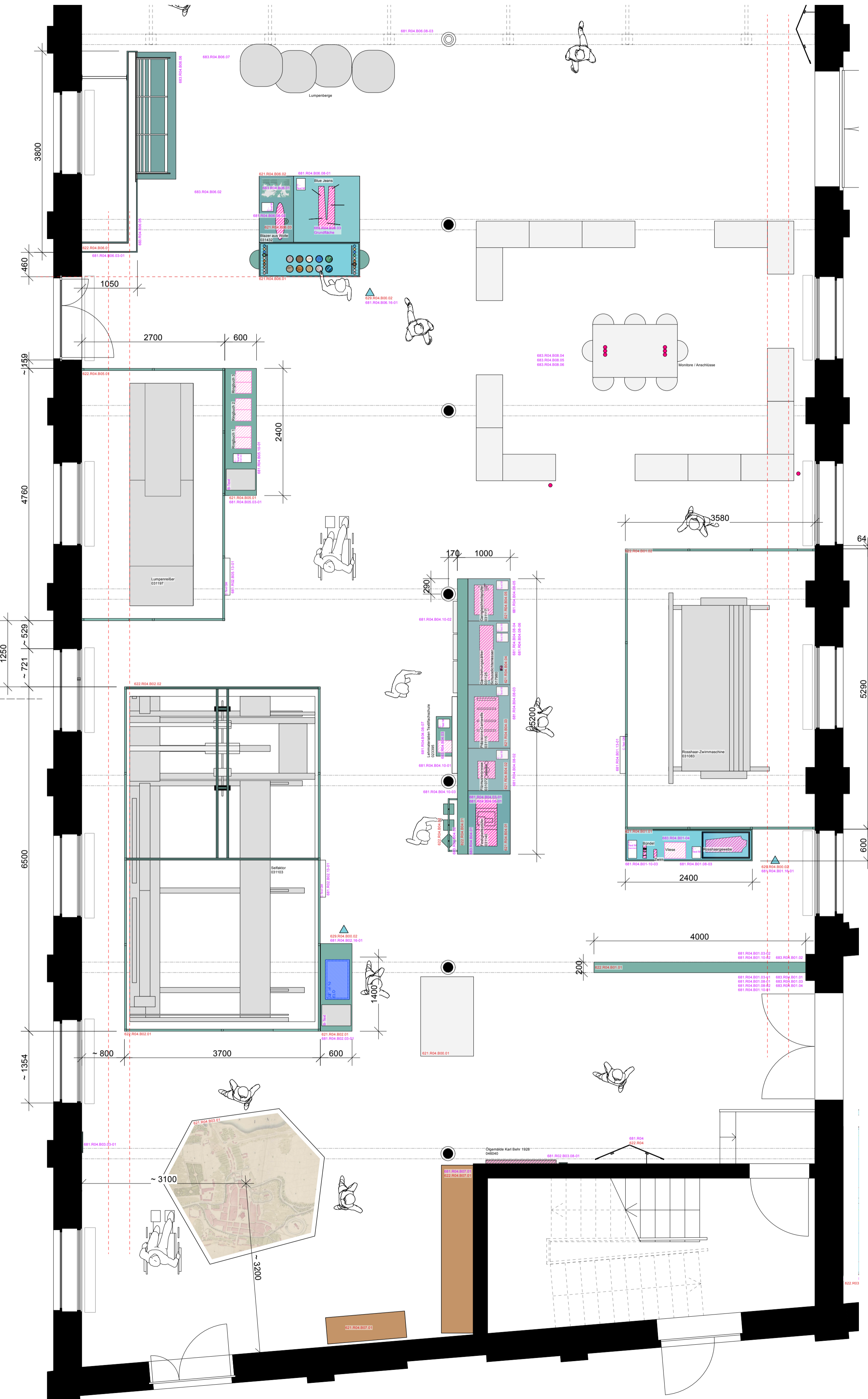
Grundriss M1:50
