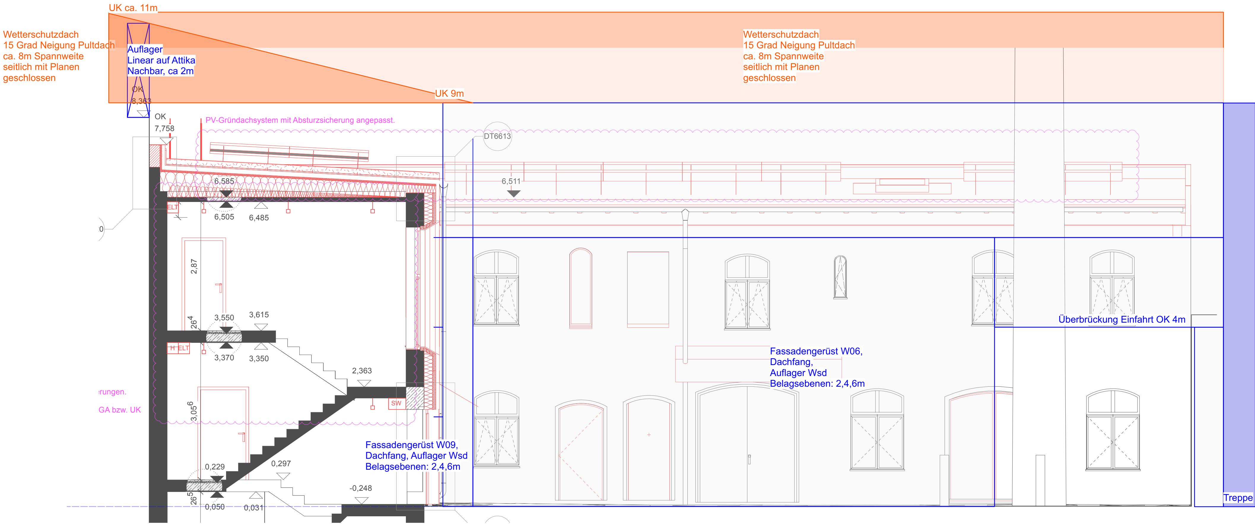
Ansicht Nord
