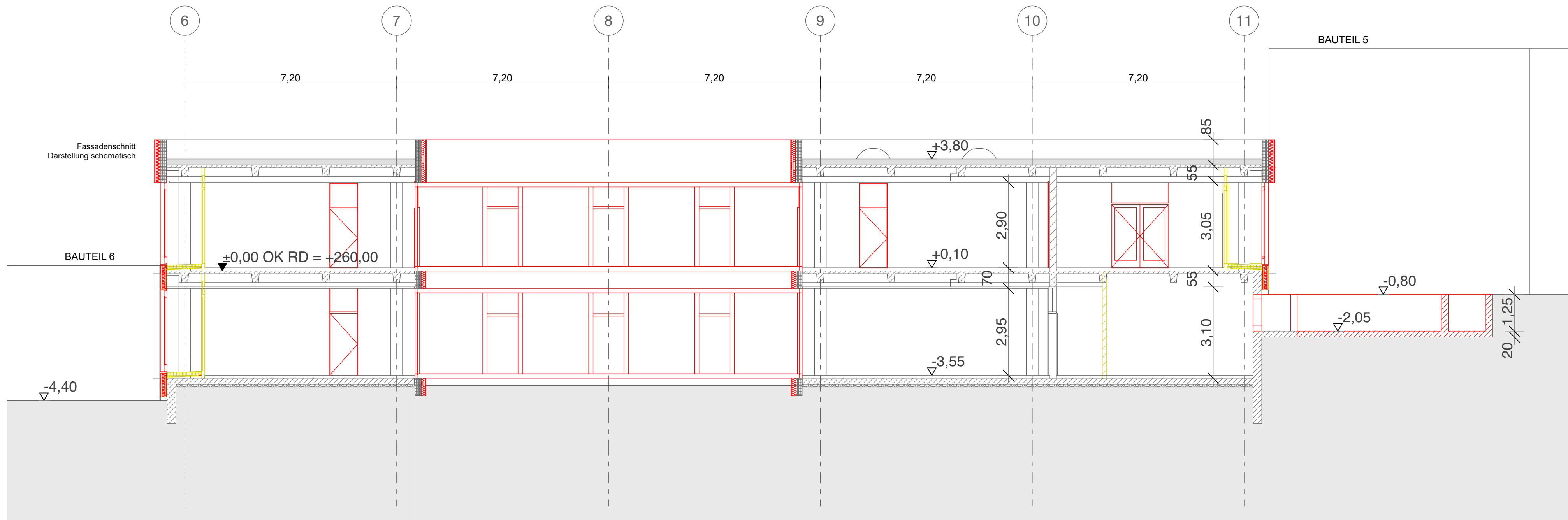
B Querschnitt 1:100
