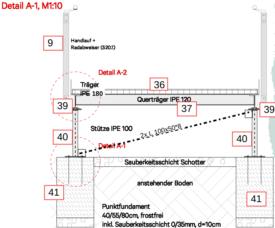
Querschnitt - Rampe, M1:25
