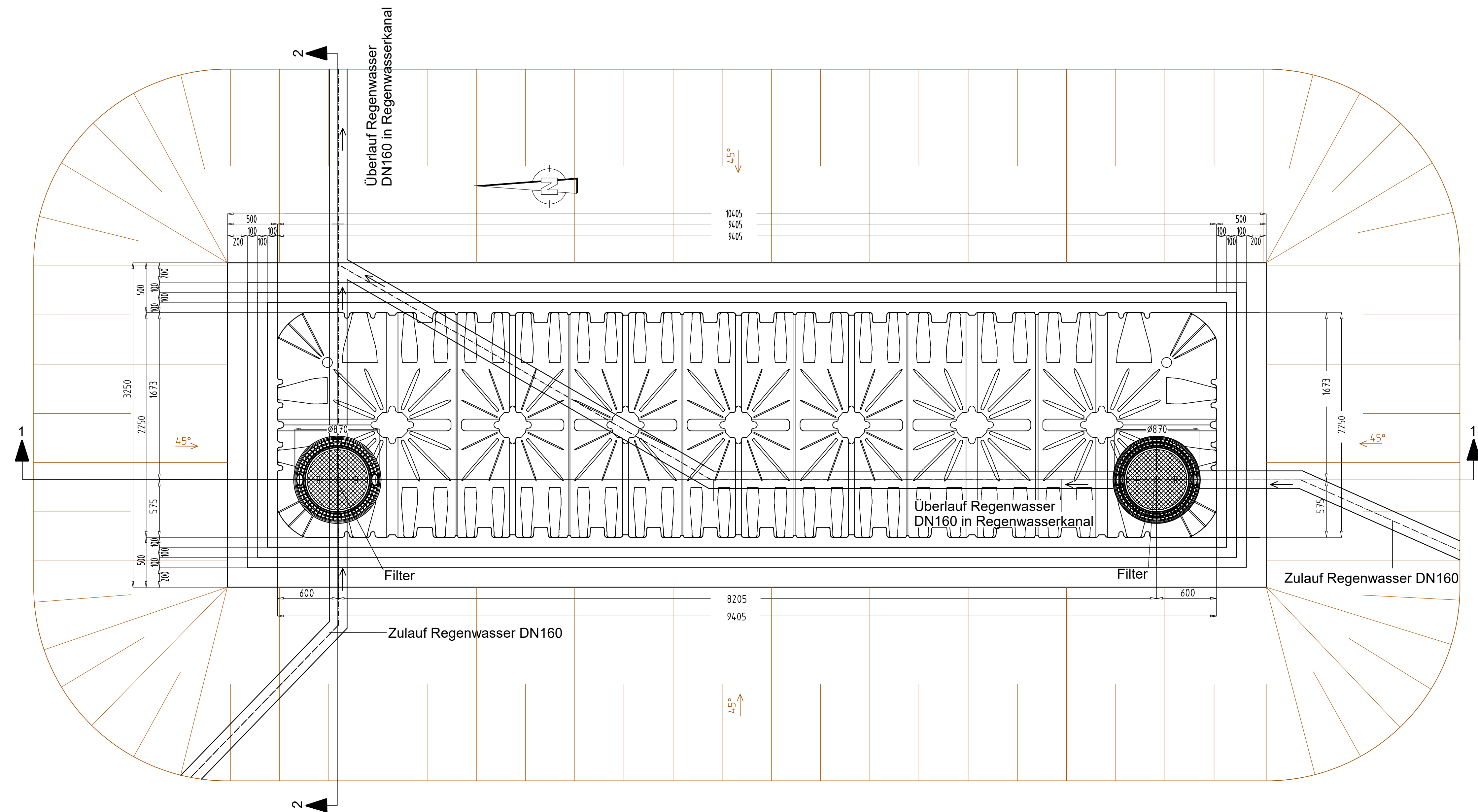
Draufsicht 1:25
