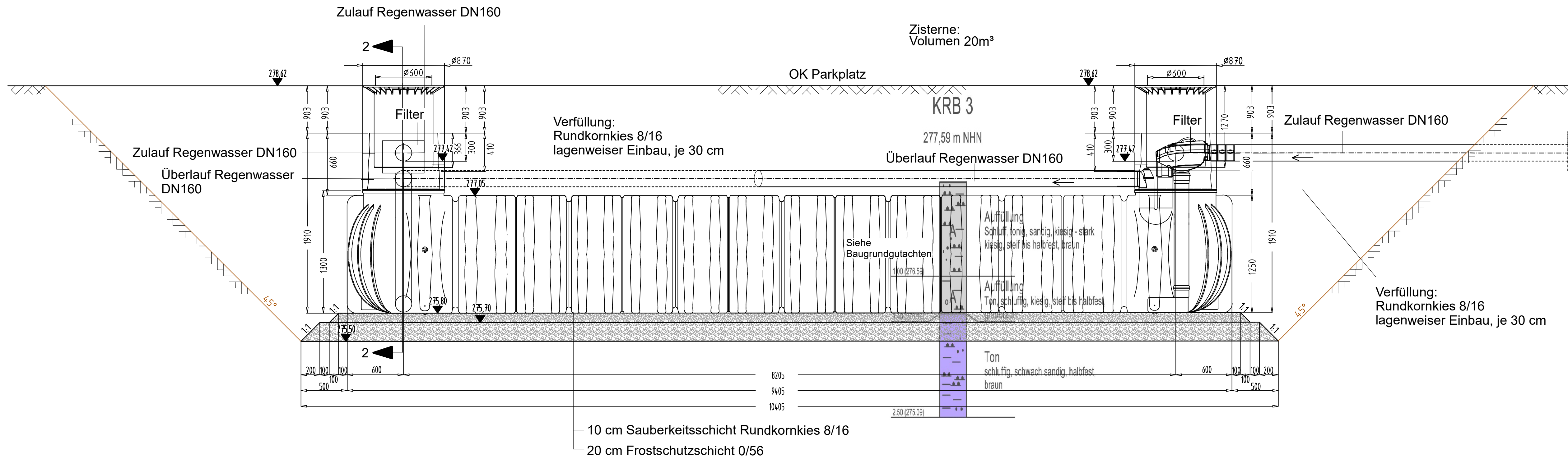
Längsschnitt 1-1 1:25
