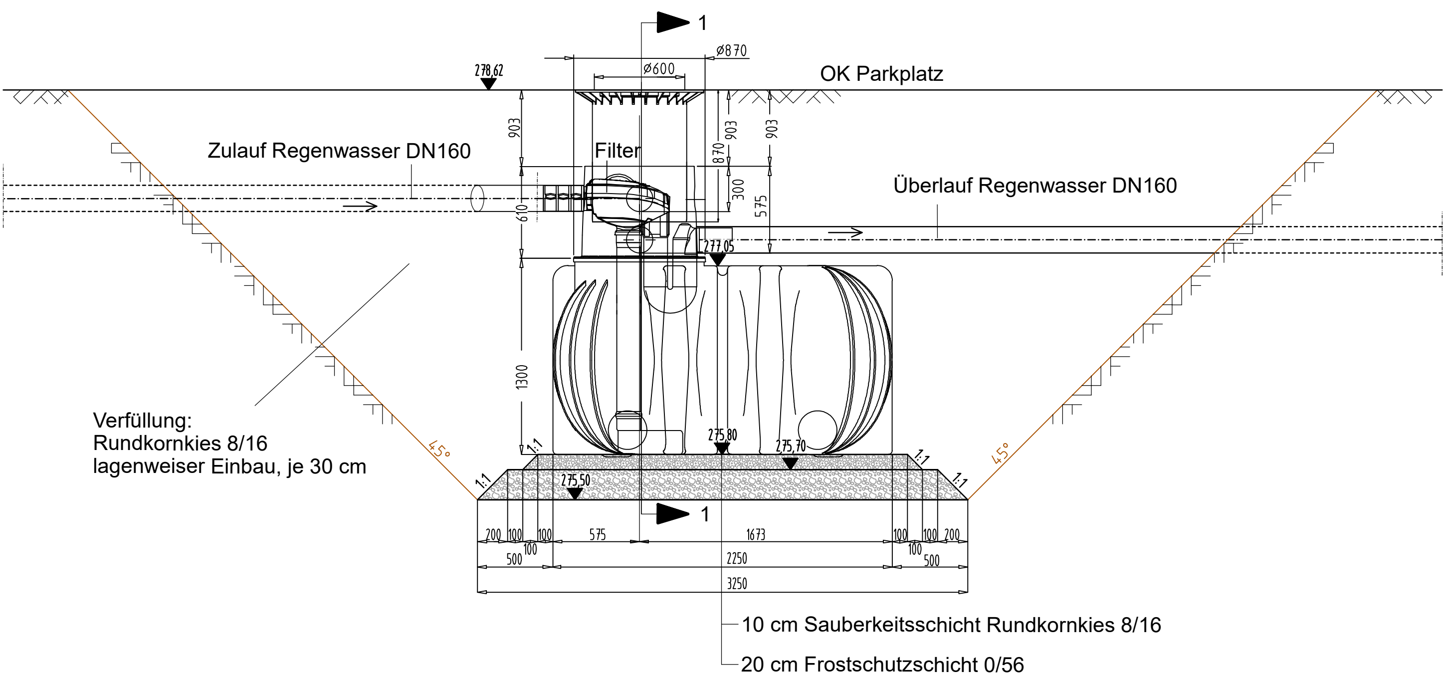
Querschnitt 2-2 1:25
