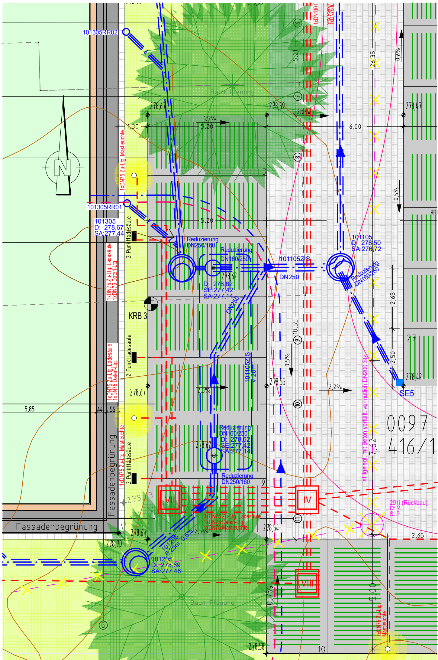
Detail Lageplan 1:100
