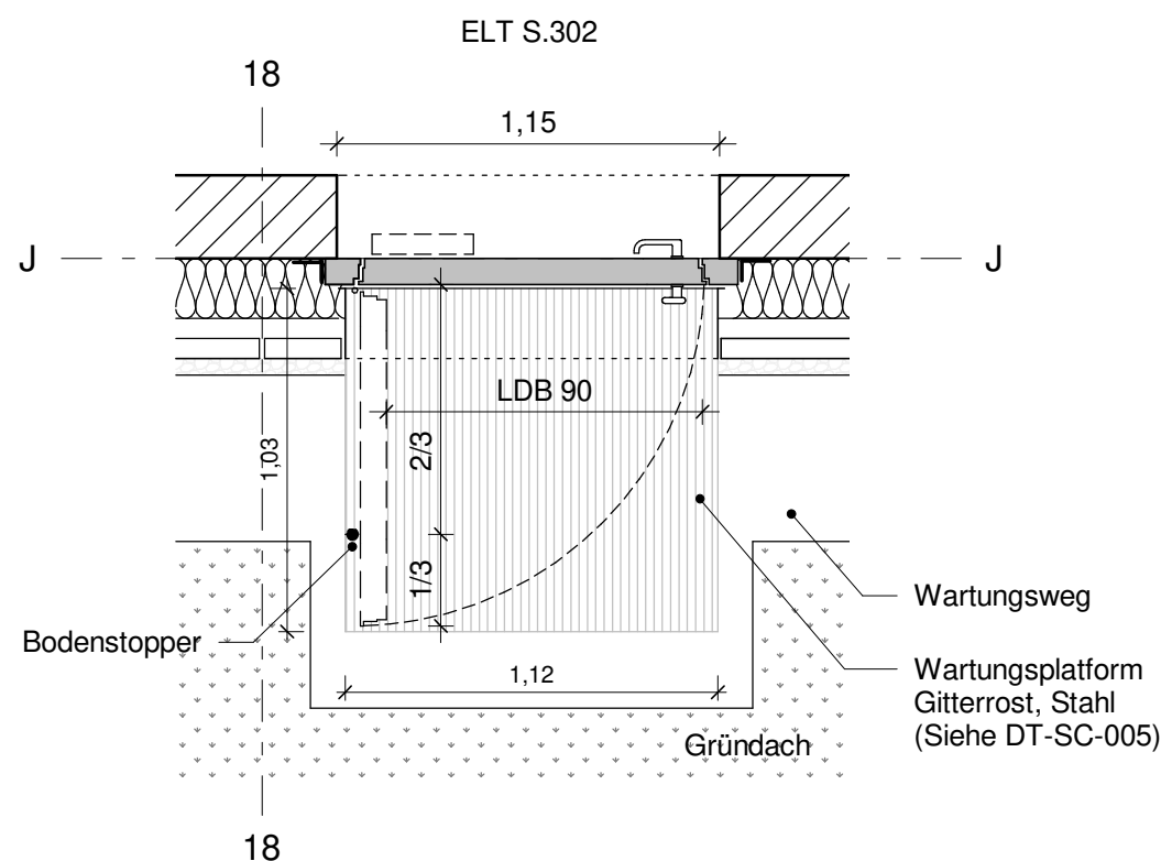
Grundriss 286
