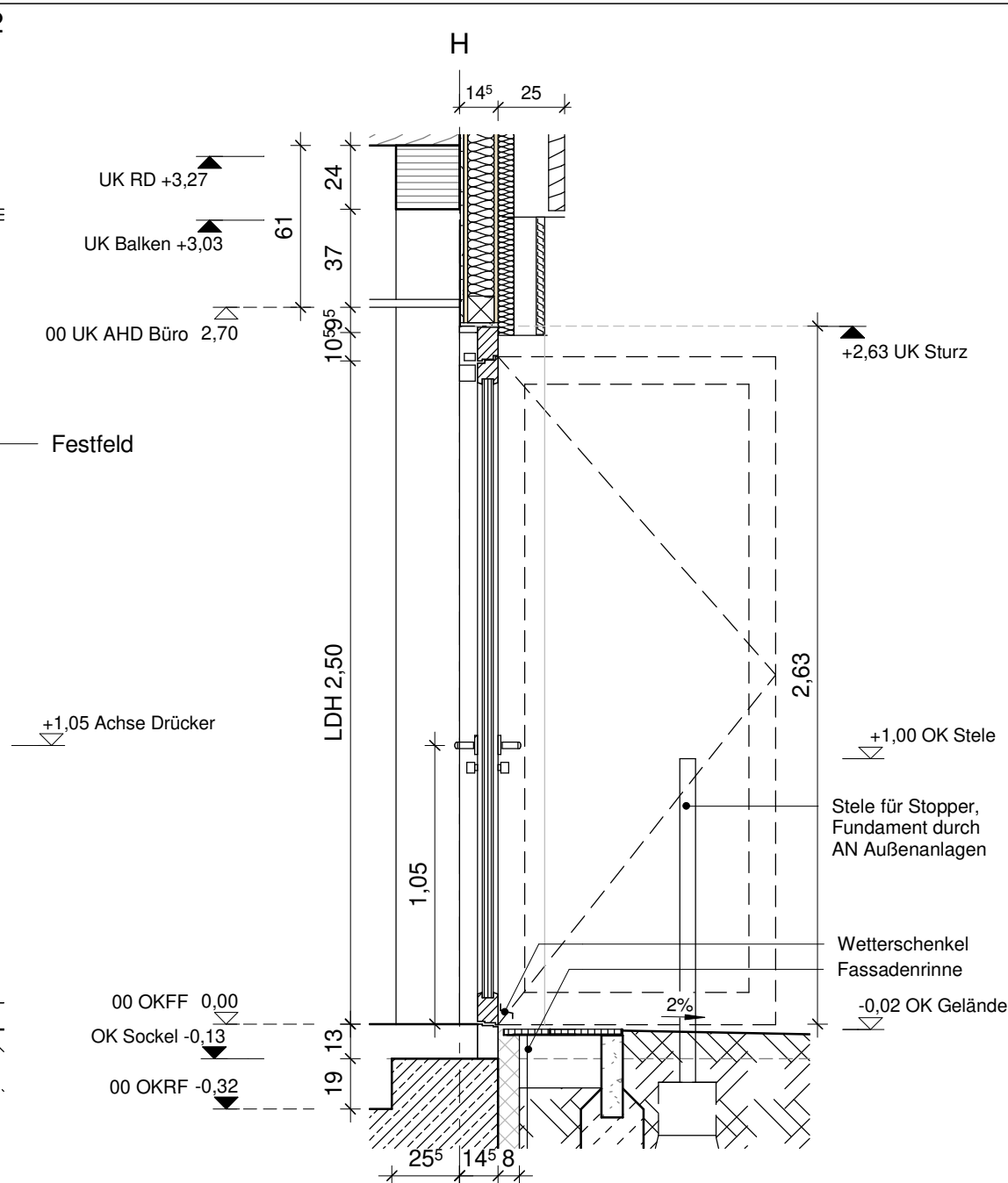
Schnitt 279
