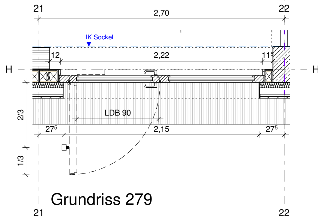
Ansicht 279
