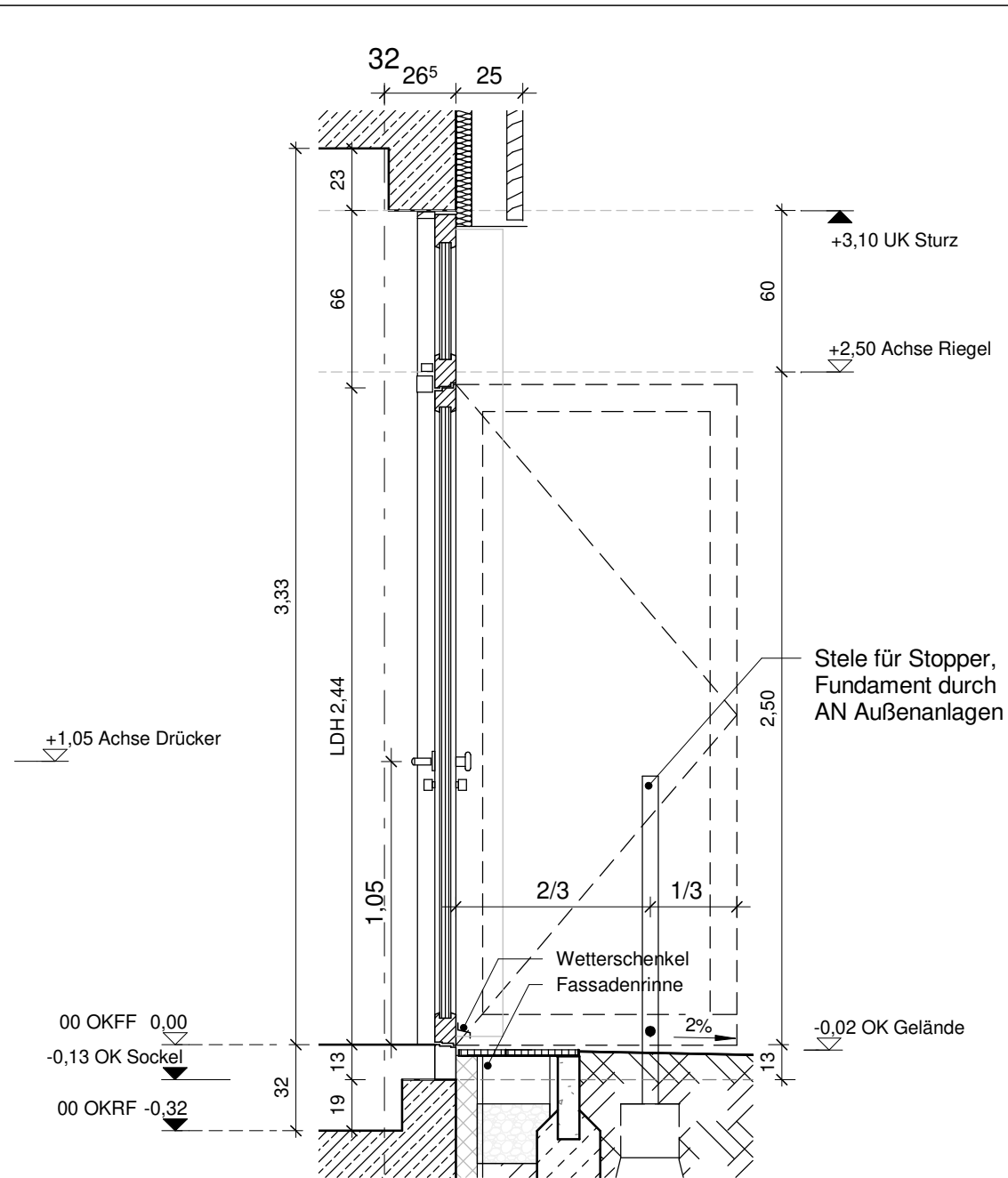
Schnitt 276
