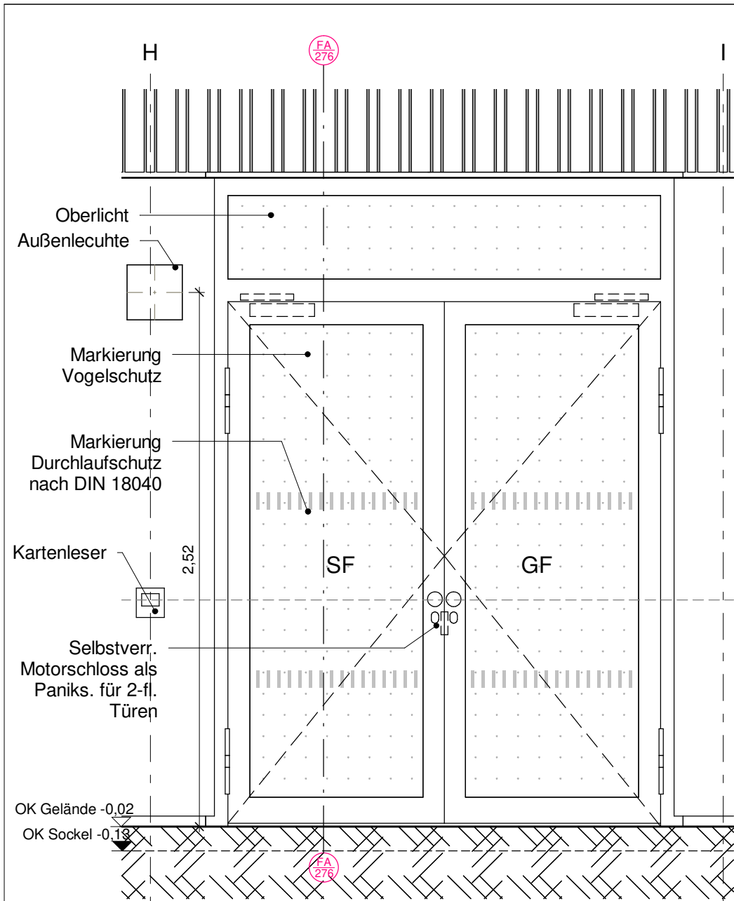
Ansicht 276
