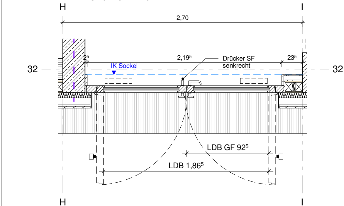
Grundriss 276
