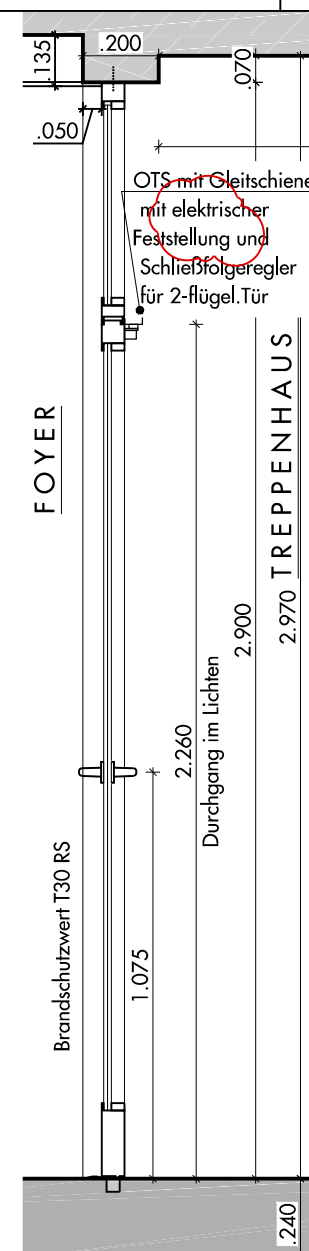
Vertikalschnitt A-A
