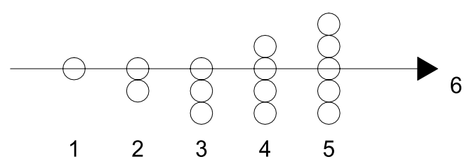
Beispielhafte Anordnung von Geräte-/Geräteverbindungsdoesen nach DIN 18015-3:2016-09
