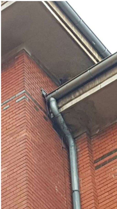
Dachauskragung
