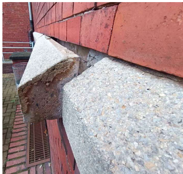
Sockelabdeckung Betonwerkstein
