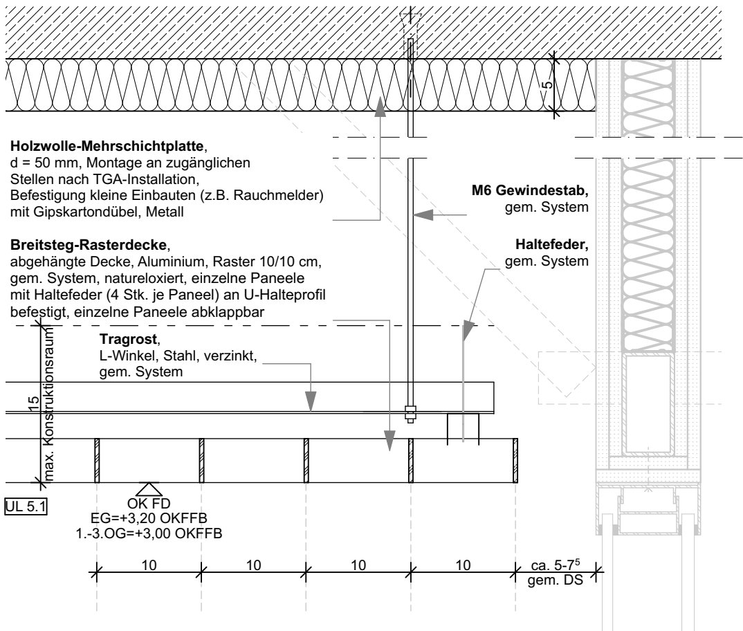
TD18 Rasterdecke, Anschluss an TB-Sturz Foyer 1.OG, Schnitt
