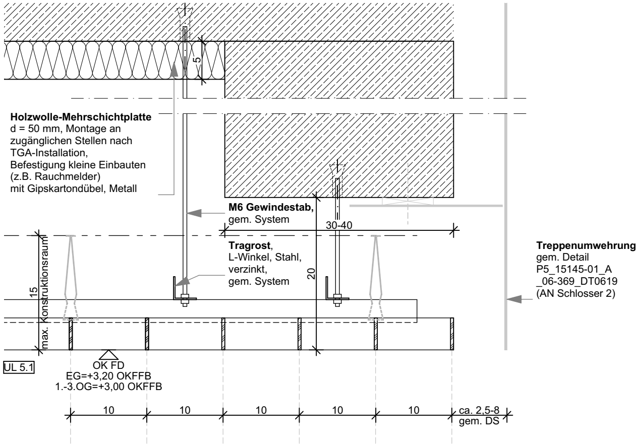
TD16 Rasterdecke, Anschluss an Unterzug, Foyer, Schnitt
