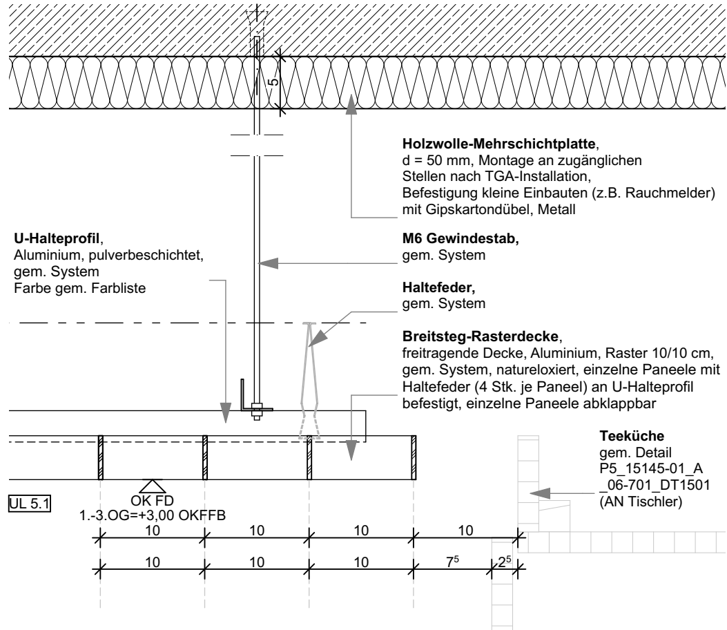
TD17 Rasterdecke, Anschluss Teeküche Foyer, Schnitt
