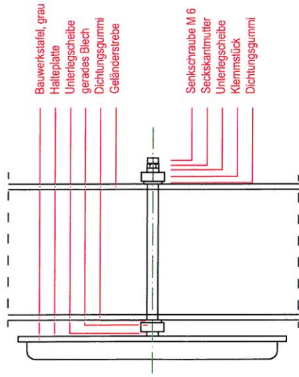
Schnitt C-C M 1:2
