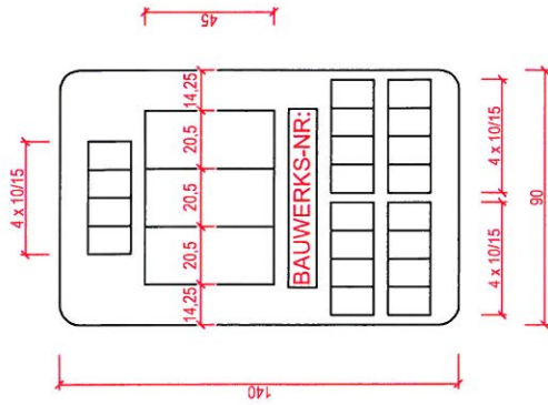
Bauwerkstafel Ansicht M 1:2
