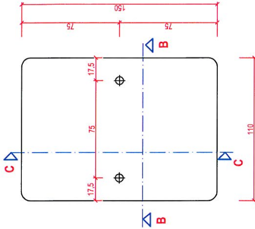
Halteblech Alu, Ansicht M 1:2
