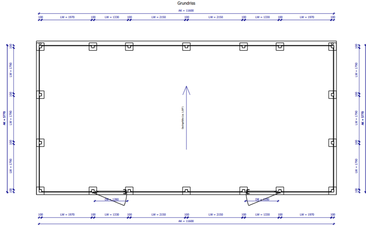
Grundriss
