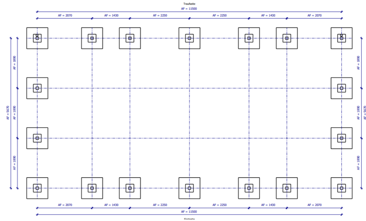
Traufseite
