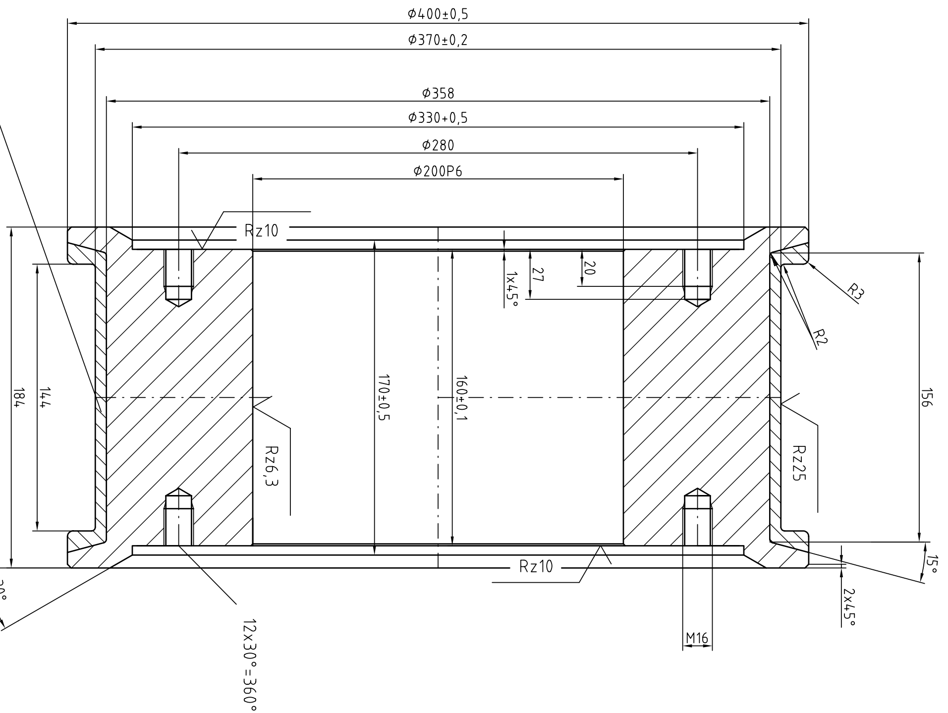
10 ✓ Rz100 (✓) Rollenkörper M1:2
