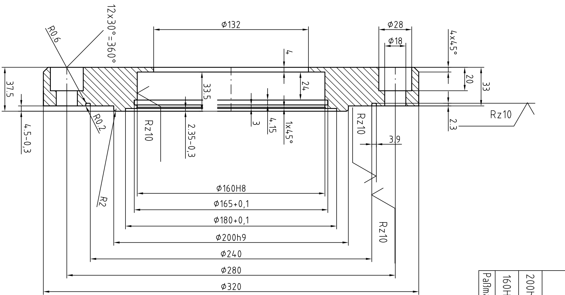
9 ✓ Rz25 (✓) Deckel M1:2
