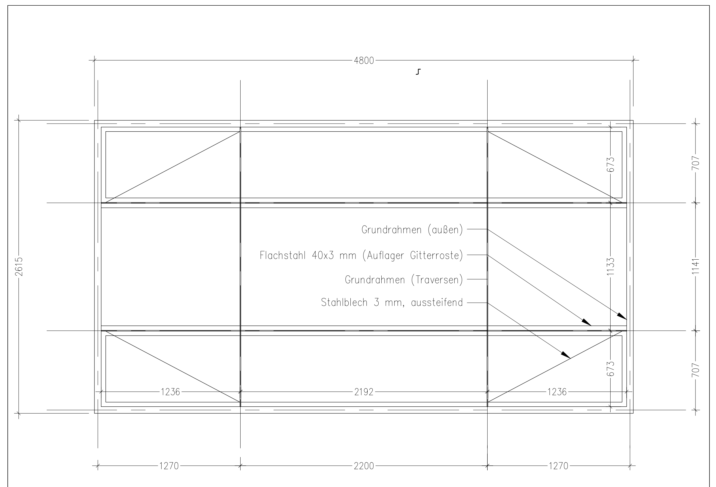
Draufsicht Schema Aufbau des Dachrahmens 1:20
