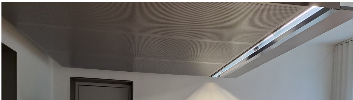
Abb. 2 Büroraum, Decke mit Metalldeckenpaneelen perforiert und Beleuchtung
