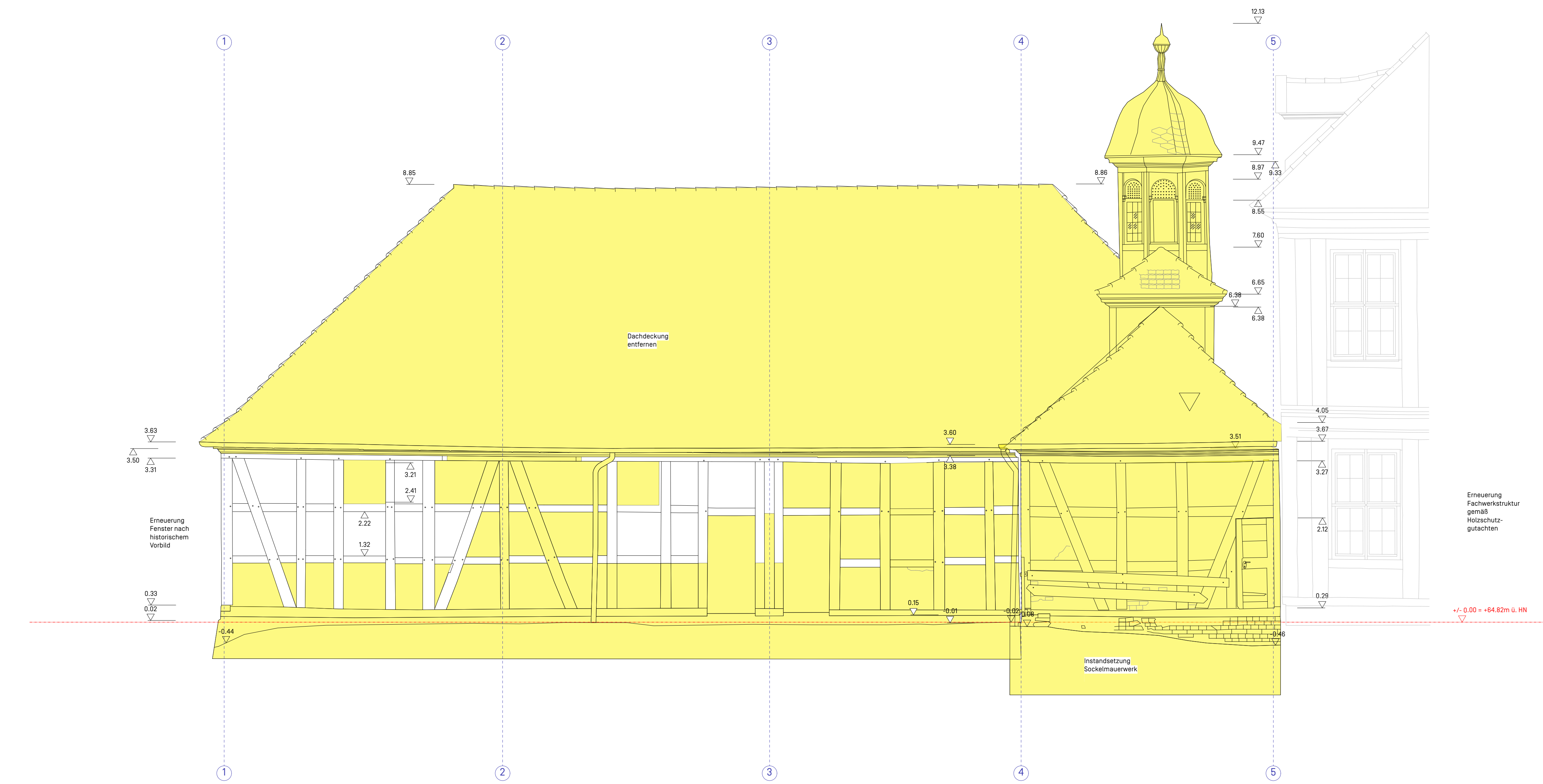
Ansicht Westen M 1:50
