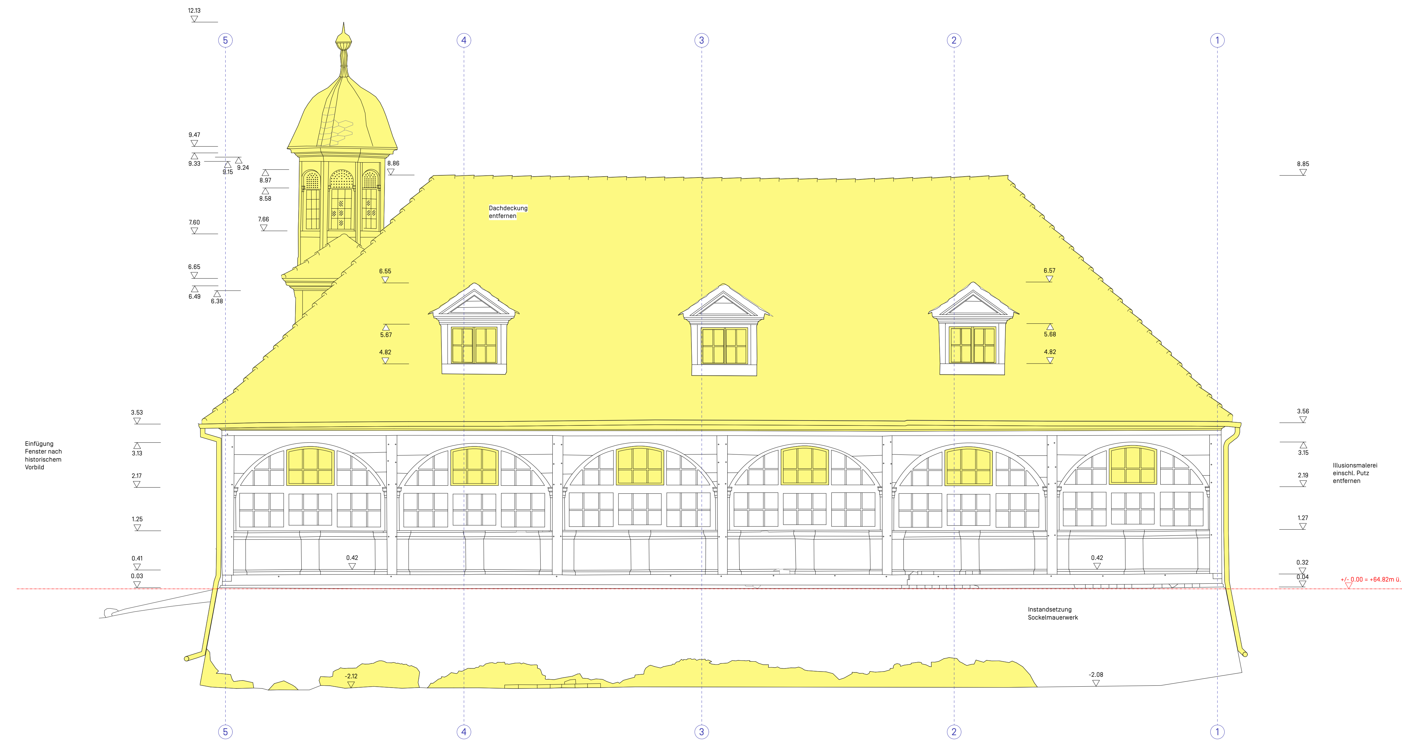
Ansicht Osten M 1:50
