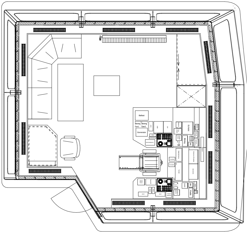
Draufsicht Steuerhaus M1:50
