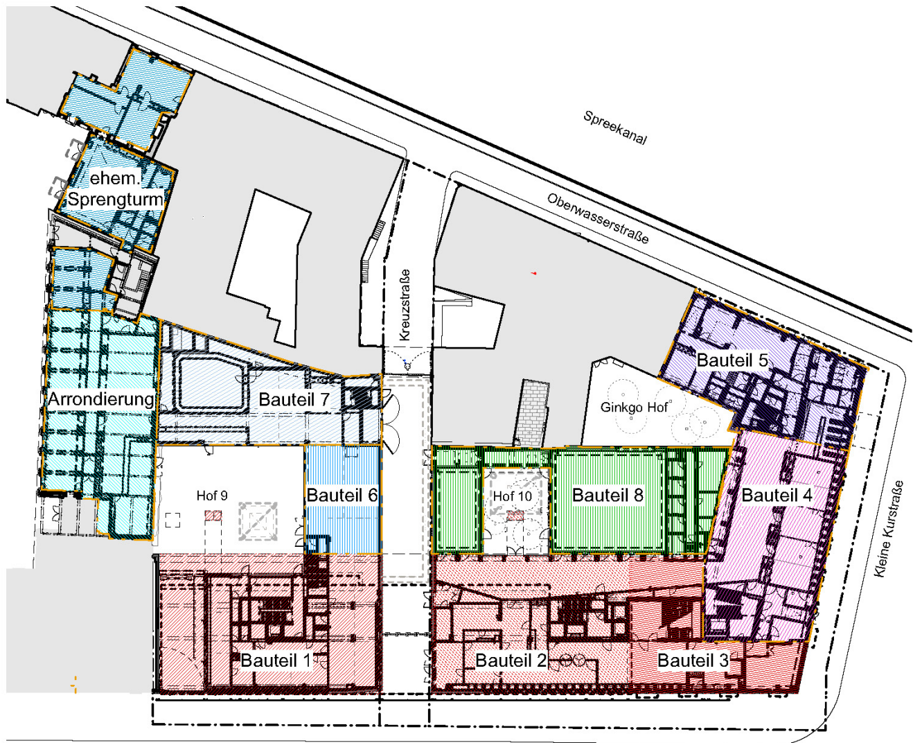
Grundriss Erdgeschoß
