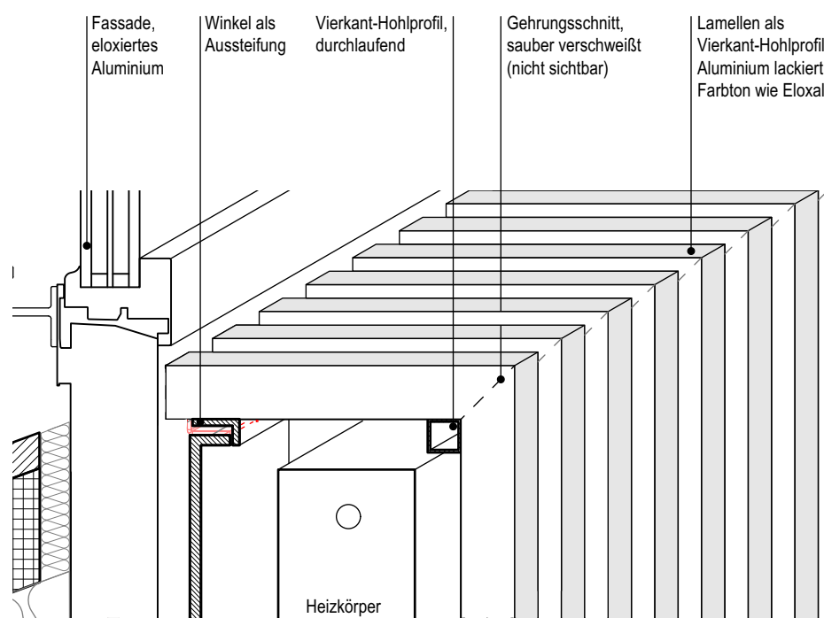
Detail oberer Anschluss geschlossen M 1:5
