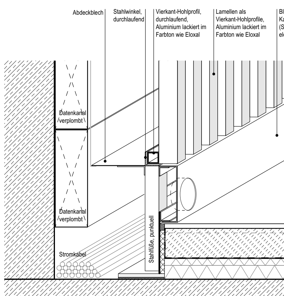
Detail Fußpunkt geschlossen M 1:5
