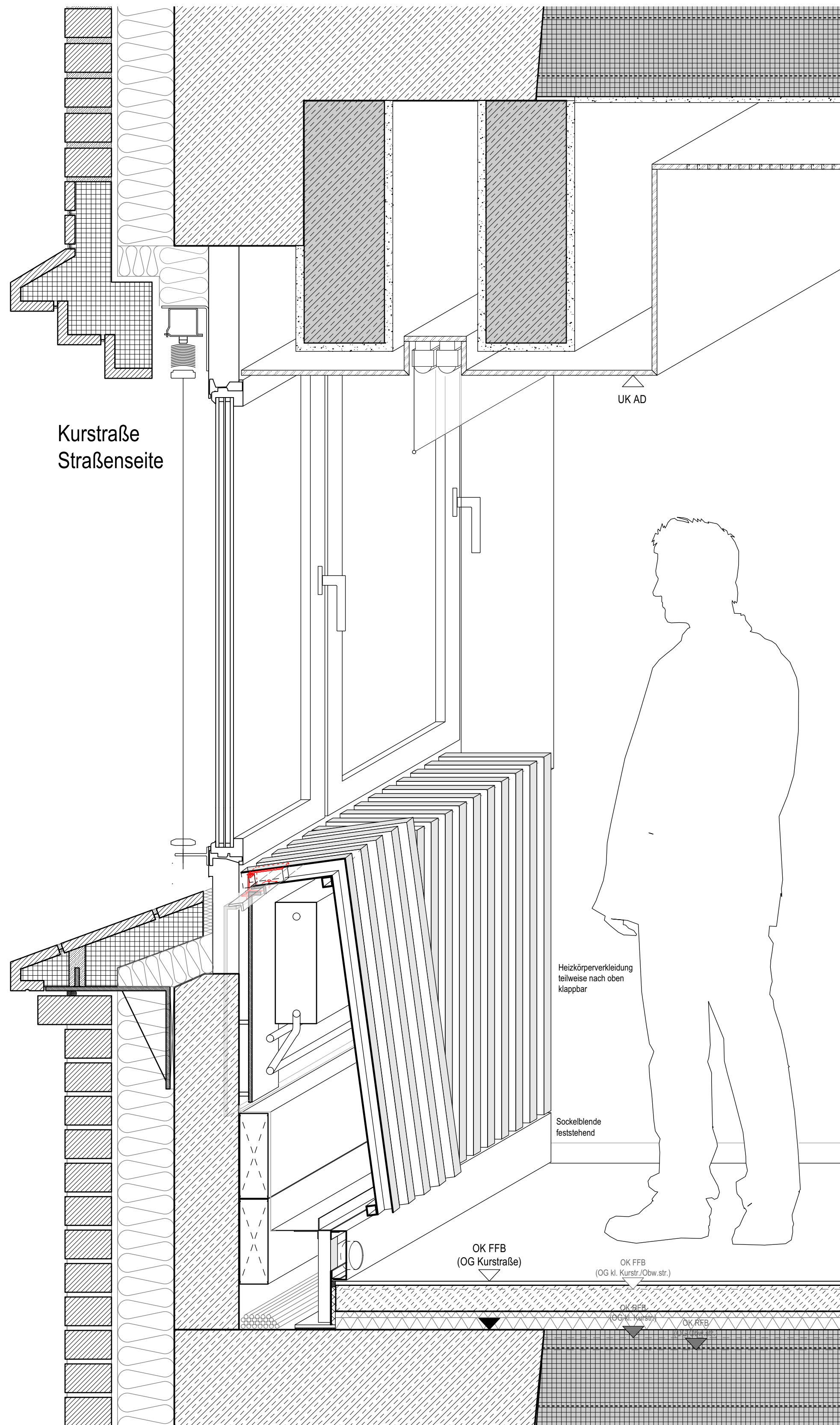
Isonometrie ohne Maßstab
