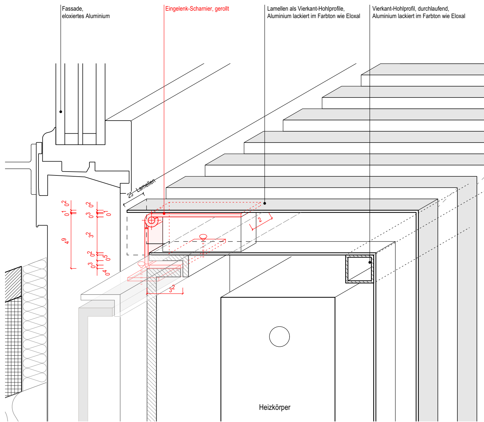
Detail Scharnier M 1:2
