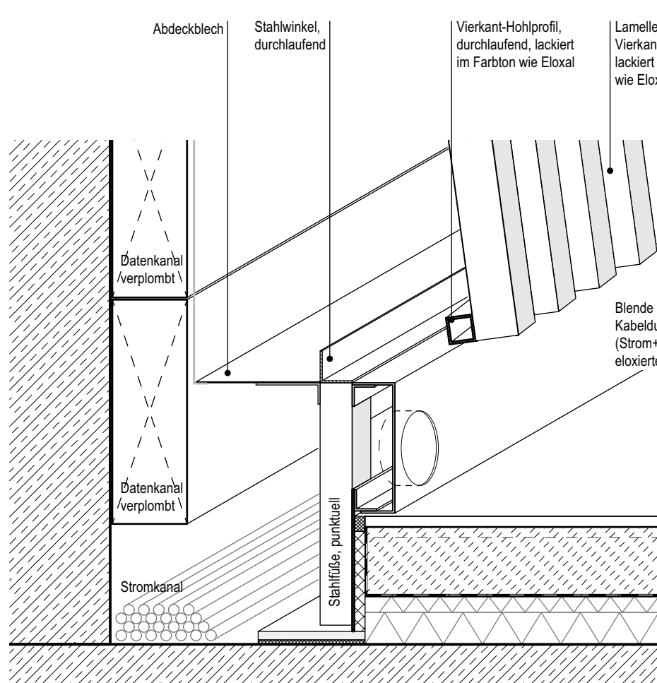
Detail Fußpunkt geöffnet M 1:5
