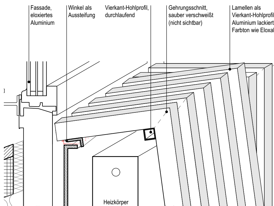
Detail oberer Anschluss geöffnet M 1:5
