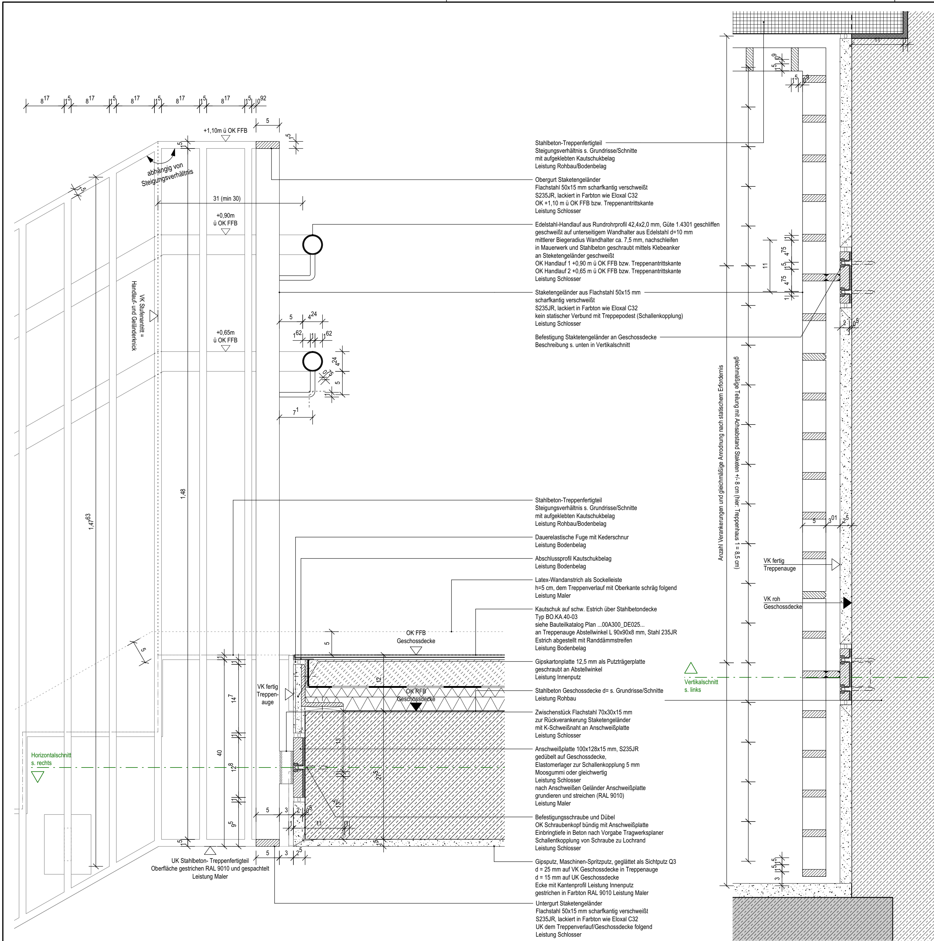
Vertikalschnitt durch Geschossdecke Horizontalschnitt durch Geschossdecke
