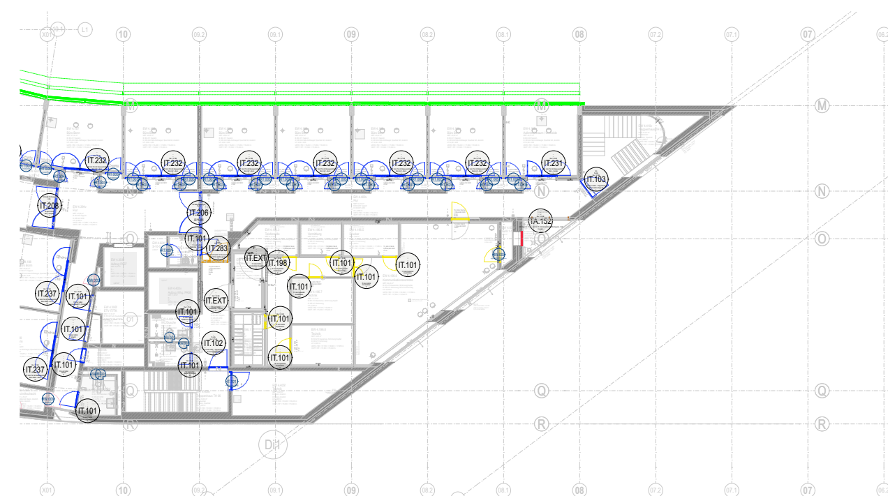
4. Obergeschoss
