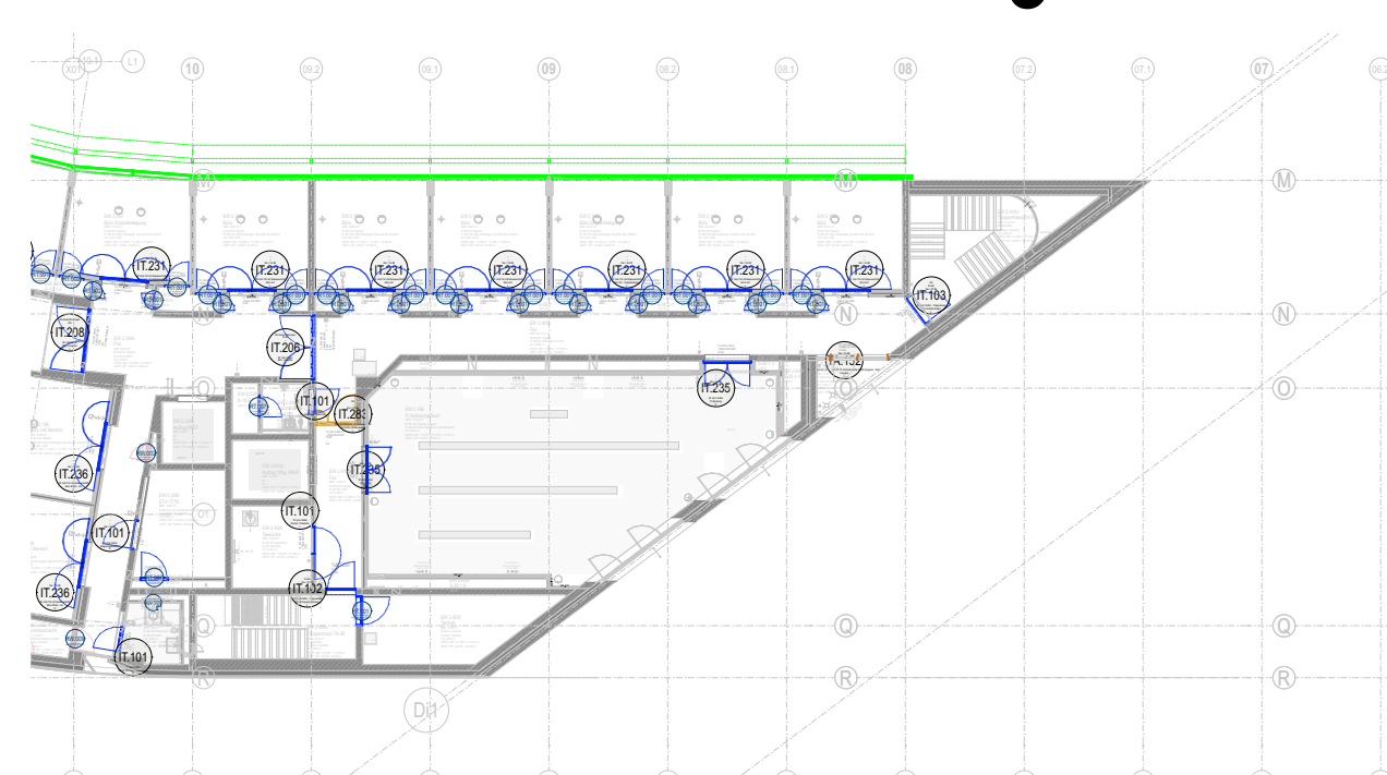
2. Obergeschoss
