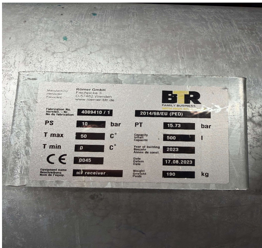
Druckluftflasche 500L (653G0001)
