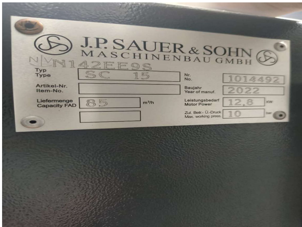
Arbeitsluftkompressor (651G0005)
