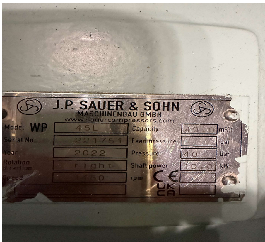
Startluftkompressor (652G0001)
