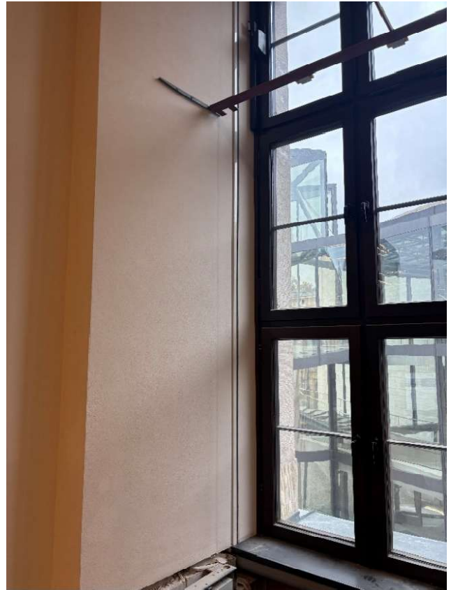
Glasfenstertüren und Alusegel, montiert und demontiert, Erstes Obergeschoss
