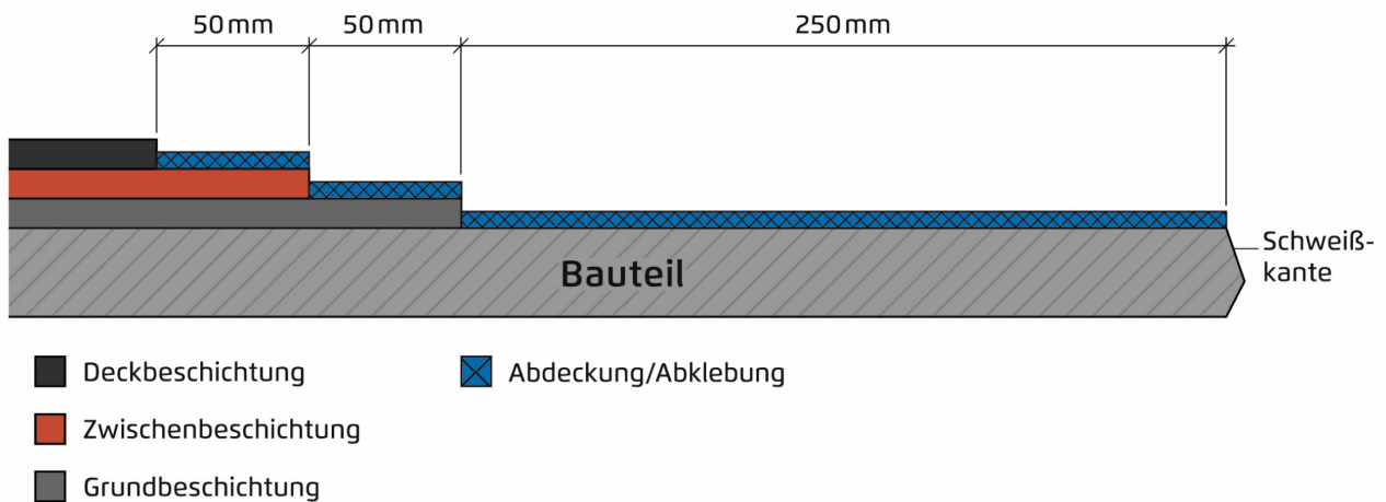
Bild A 1: Schematische Darstellung der Ausführung der Korrosionsschutzbeschichtung im Bereich von Baustellenschweißstößen bei Wärmeeinflusszonen nach (46)
