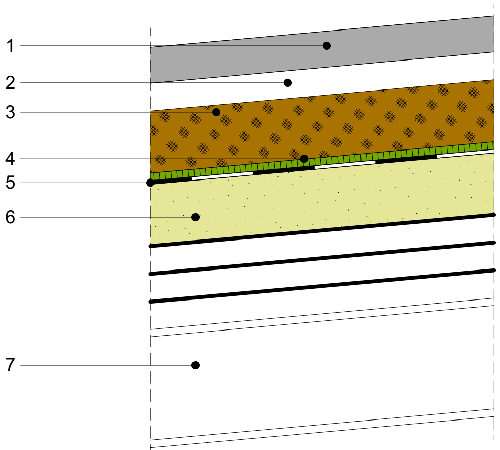
Schnitt Dachaufbau
