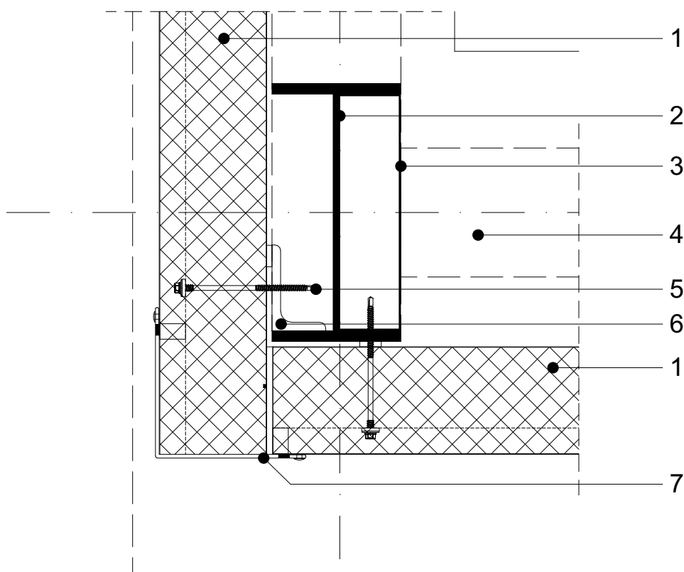
Grundriss Türanschluss
