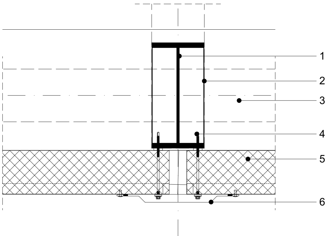
Grundriss Wandpaneelübergang
