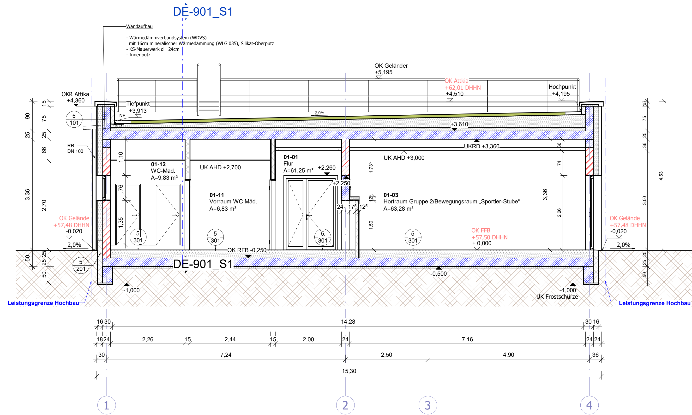
Schnitt A-A M 1 : 50
