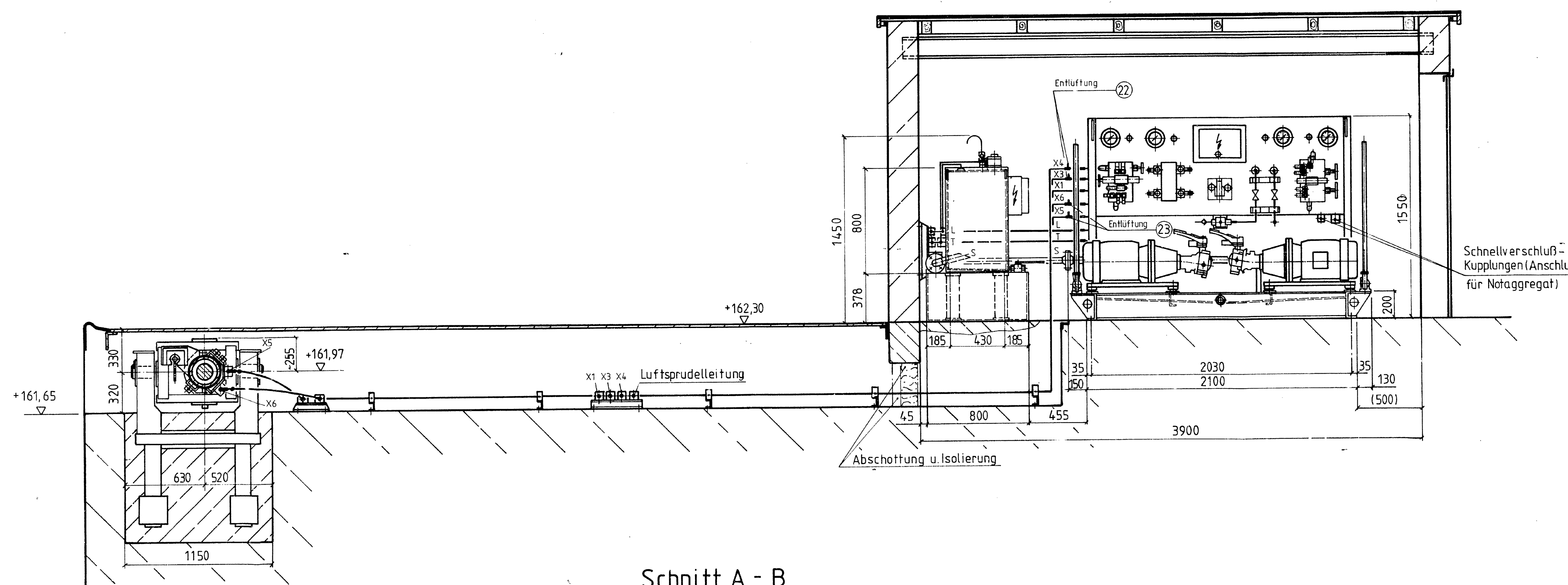
Schnitt A-B
