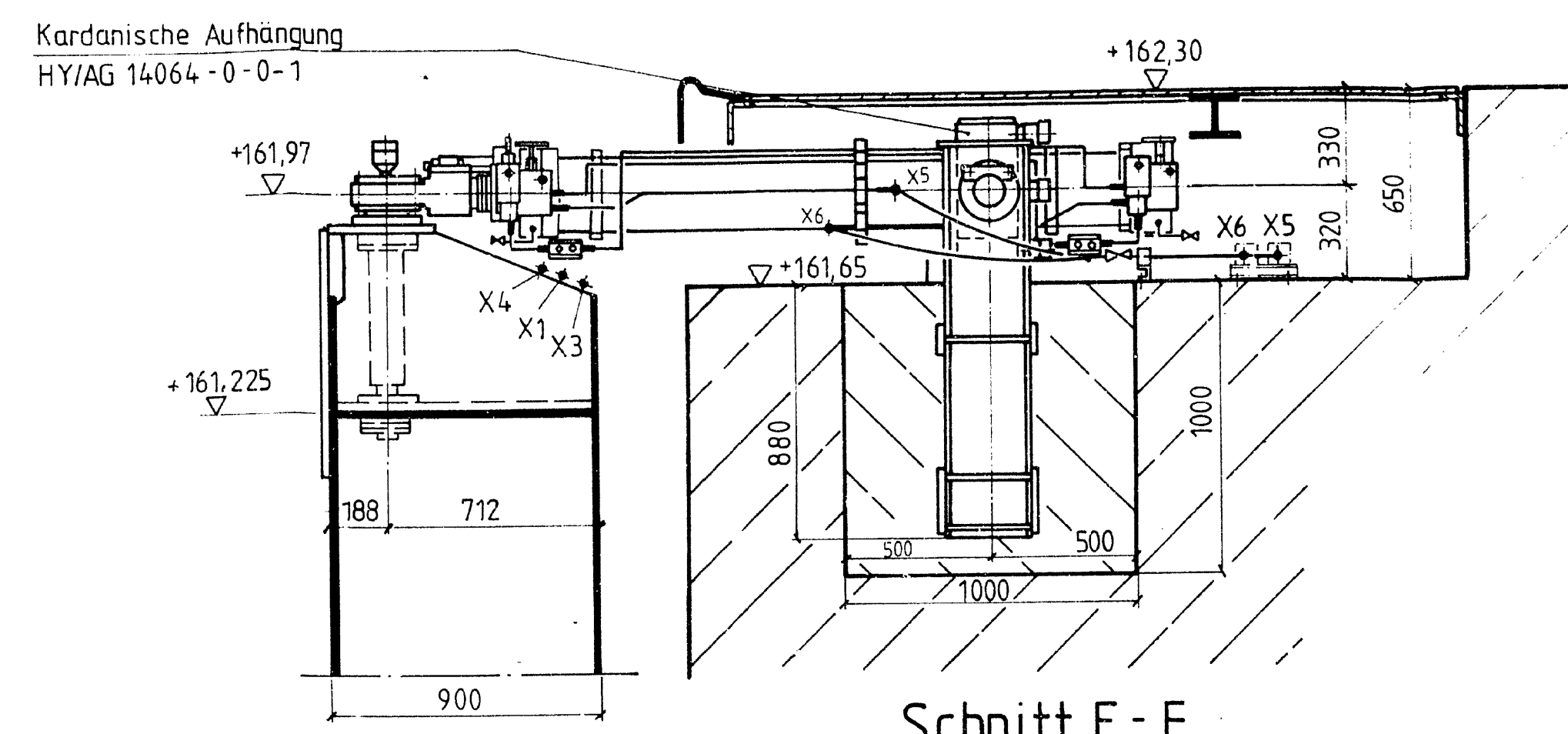
Schnitt E-F
