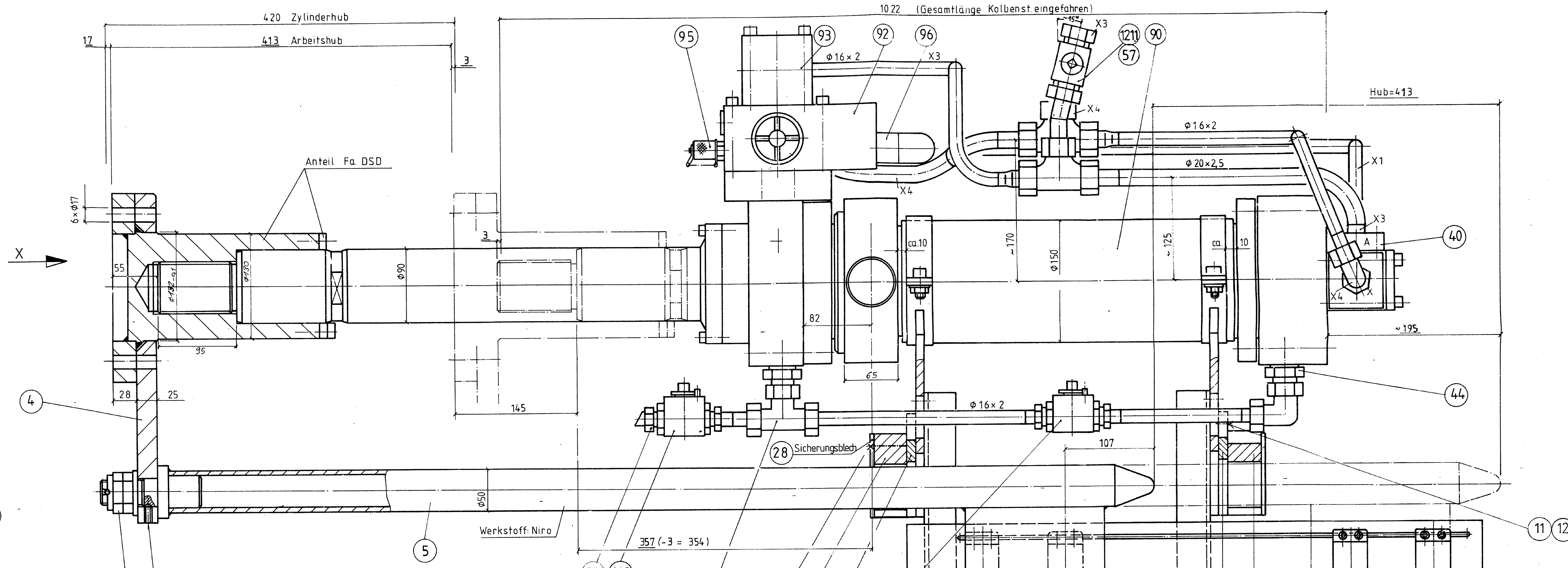
Schnitt A-B
