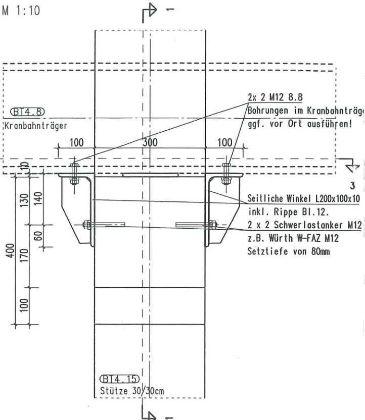
Schnitt 2-2
