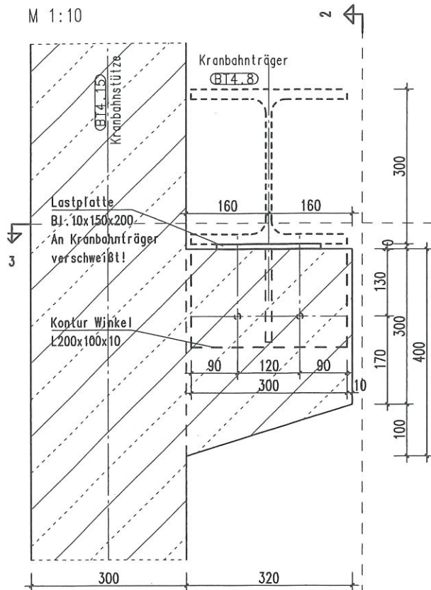
Schnitt 1-1
