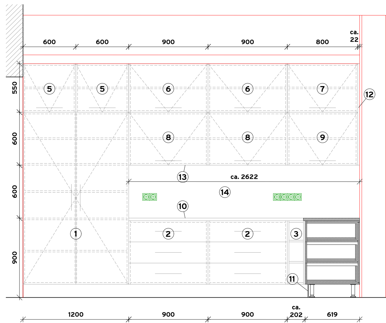
Ansicht 1
