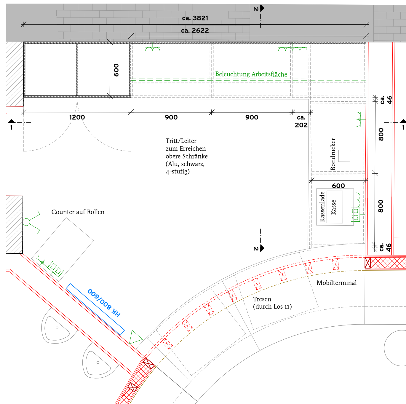
Grundriss
