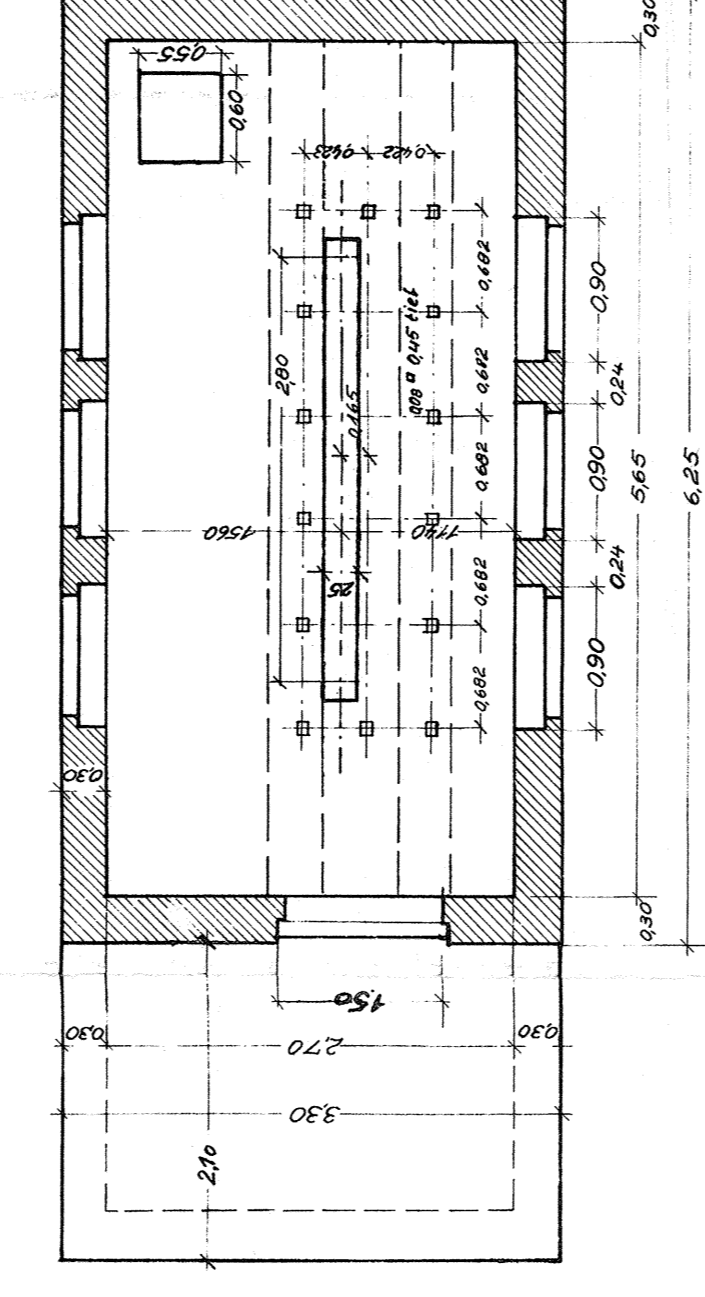
Schnitt B-B M. 1:50
