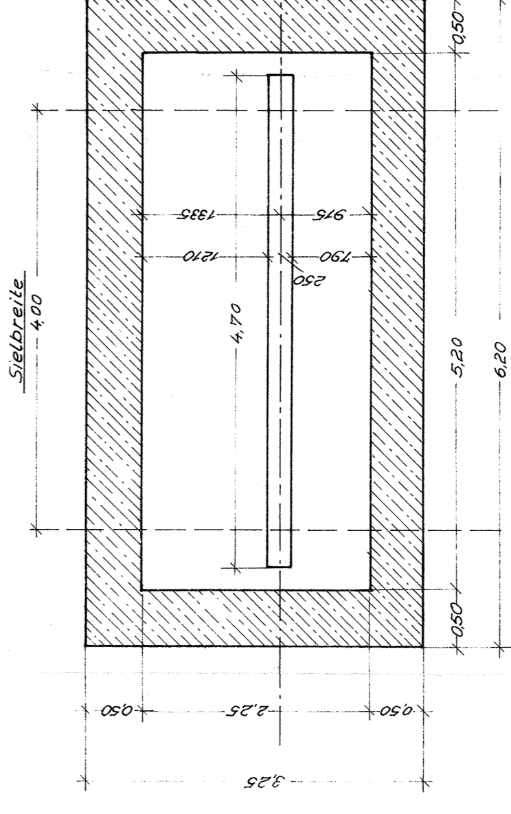
Schnitt C-C M. 1:50
