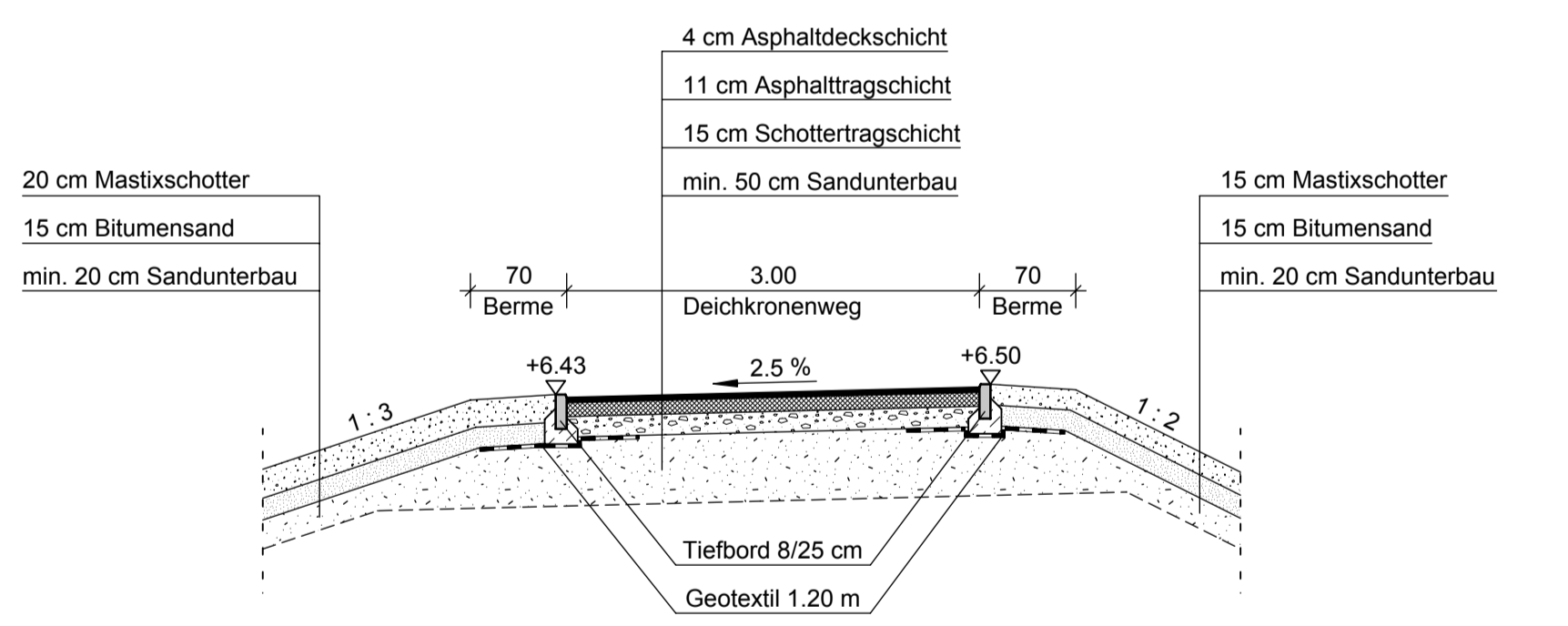
Detail Deichkronenweg M. 1 : 50
