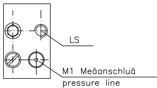
Ansicht X
