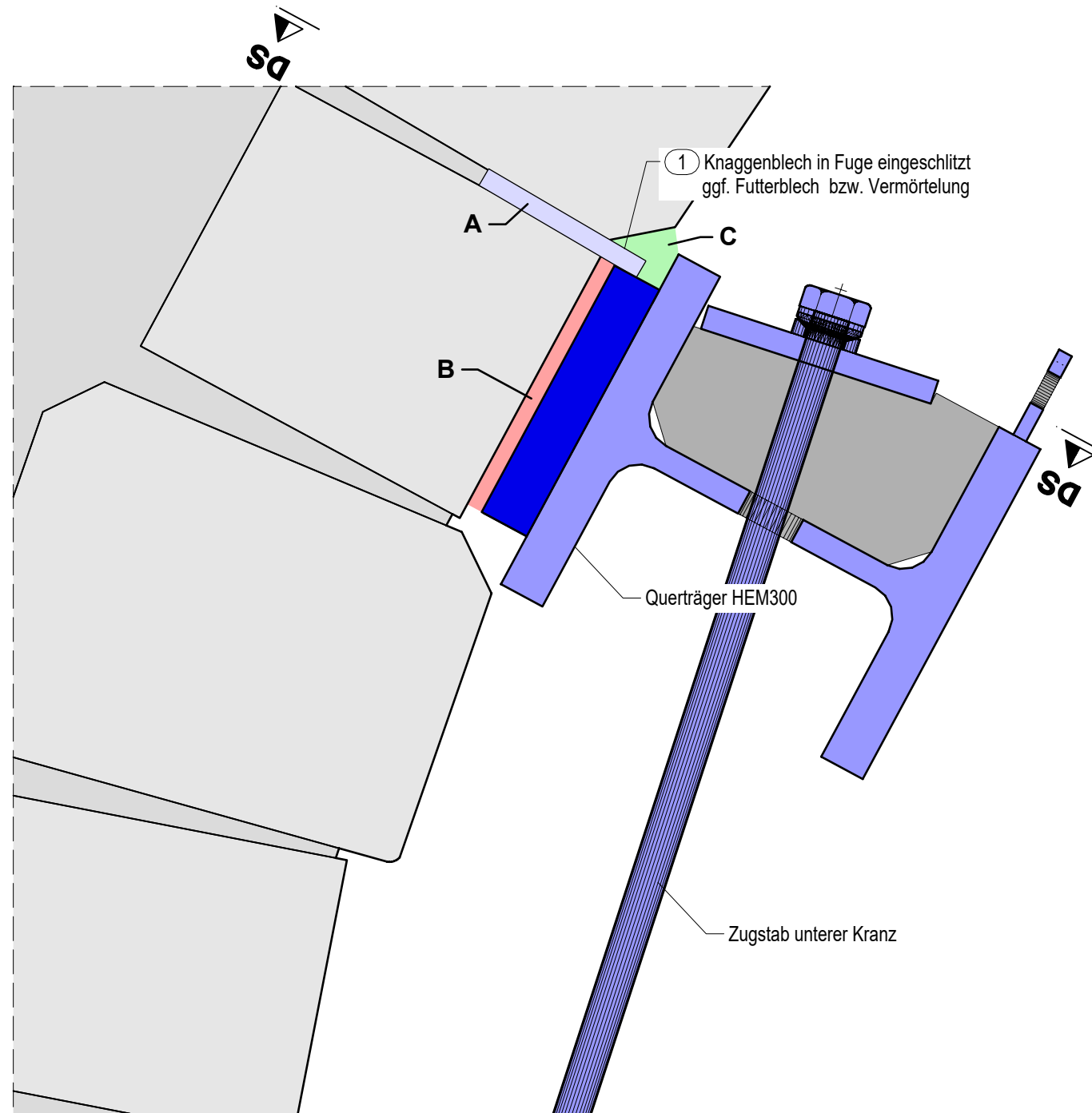
Draufsicht DS - DS ohne Maßstab
