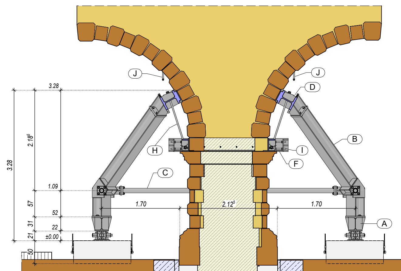
Schnitt 1 - 1
