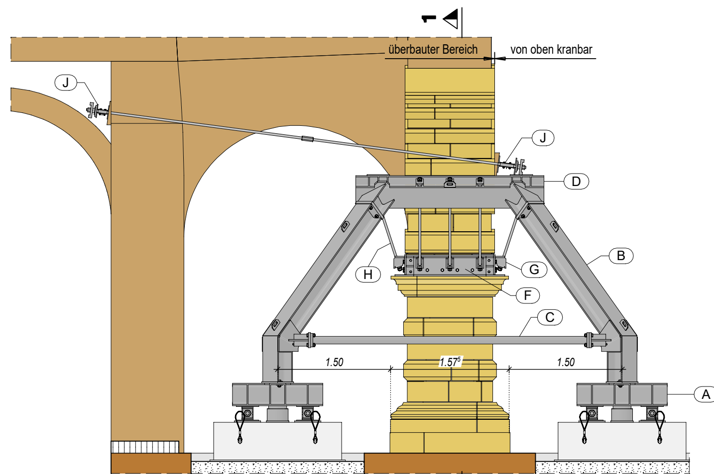
Ansicht Süden
