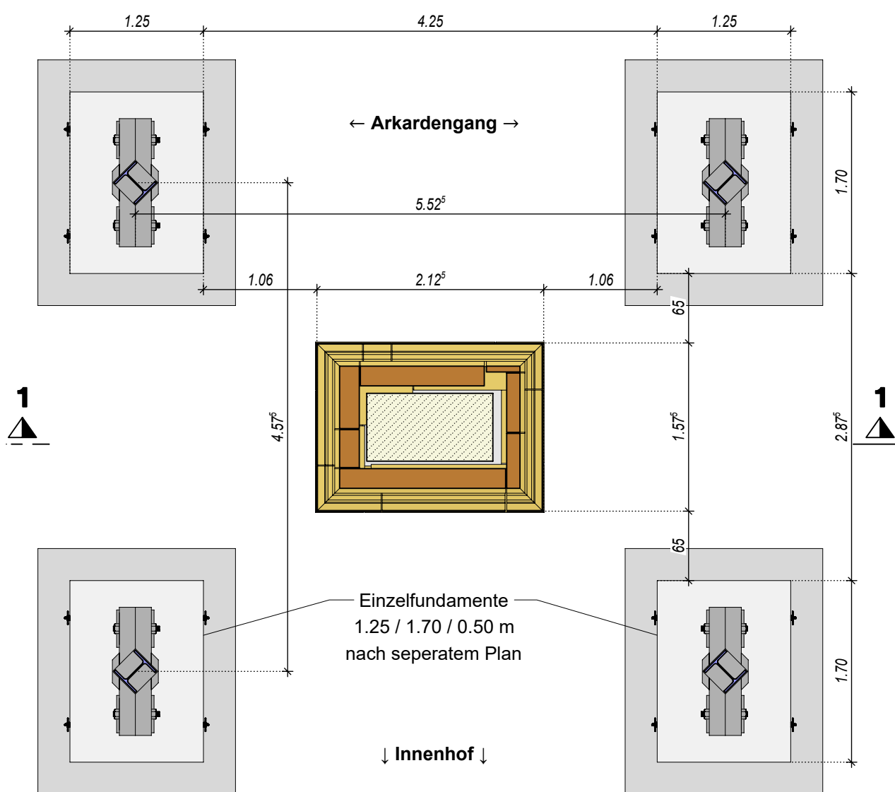
Grundriss Fundamente und Auflagerpunkte
