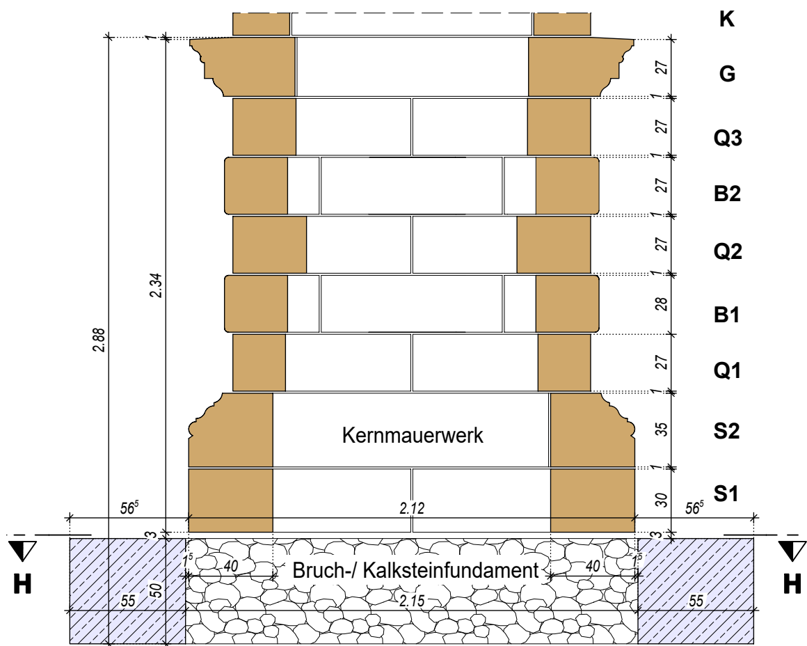
Schnitt V - V M = 1:25
