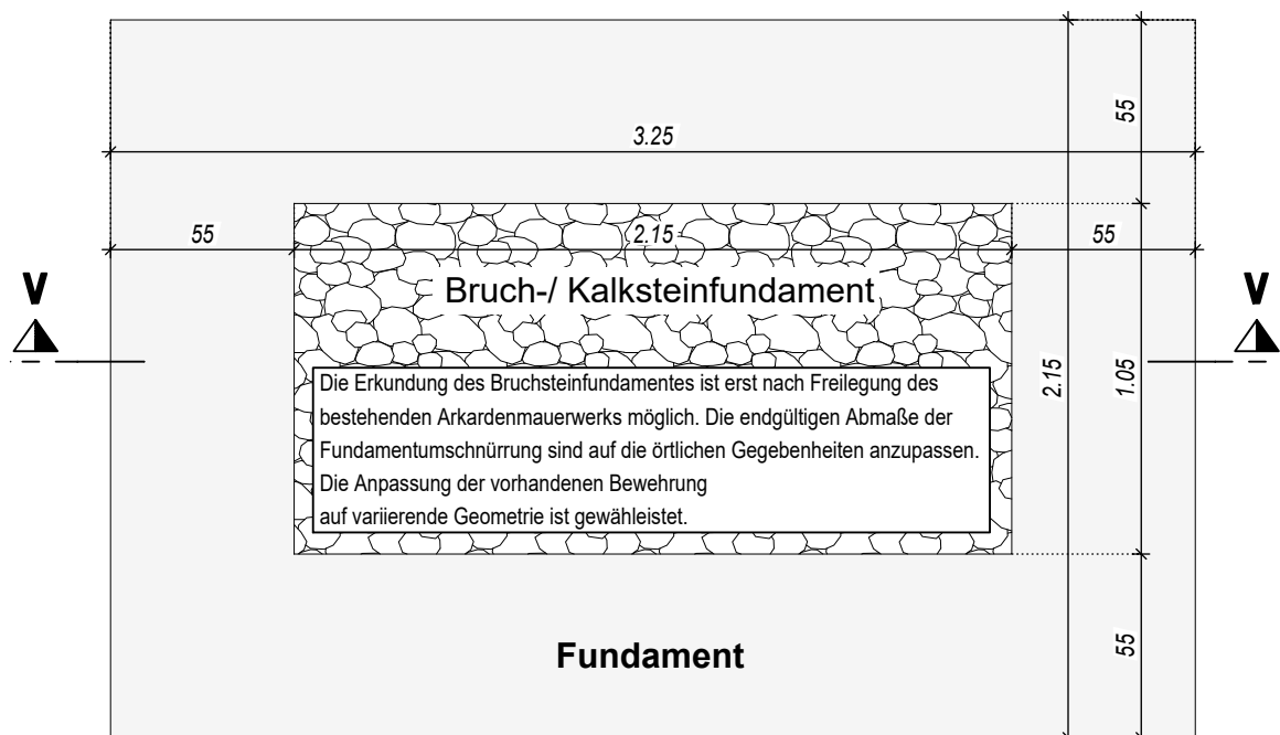
Schnitt H - H M = 1:25
