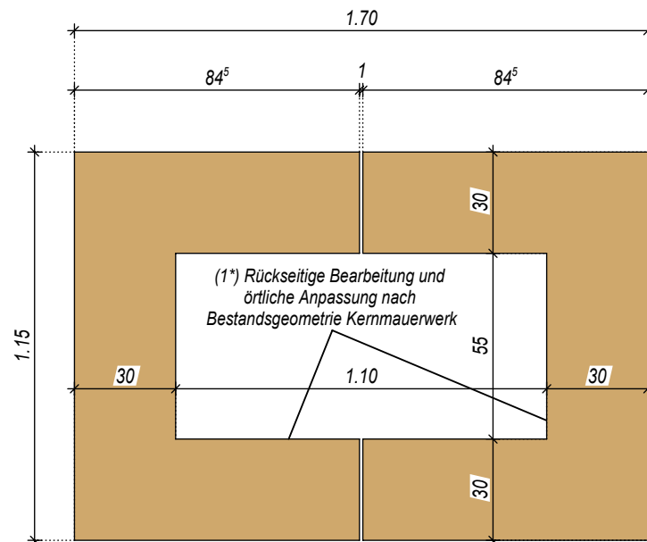
Schicht Q3 - Q3 M = 1:20 Quadermauerwerk - Ausführung 1x
