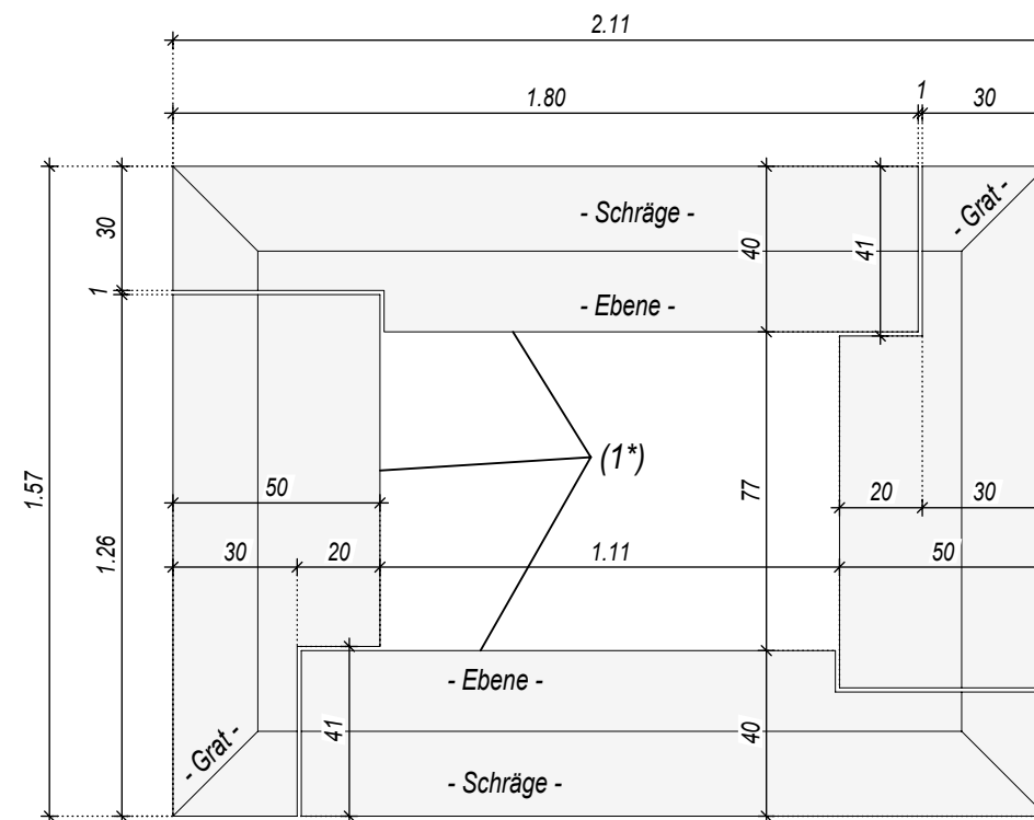
Schicht G - G Draufsicht M = 1:20 Kämpfergesims - Ausführung 1x
