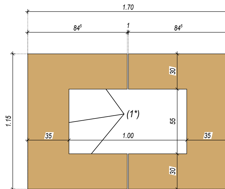
Schicht Q2 - Q2 M = 1:20 Quadermauerwerk - Ausführung 1x
