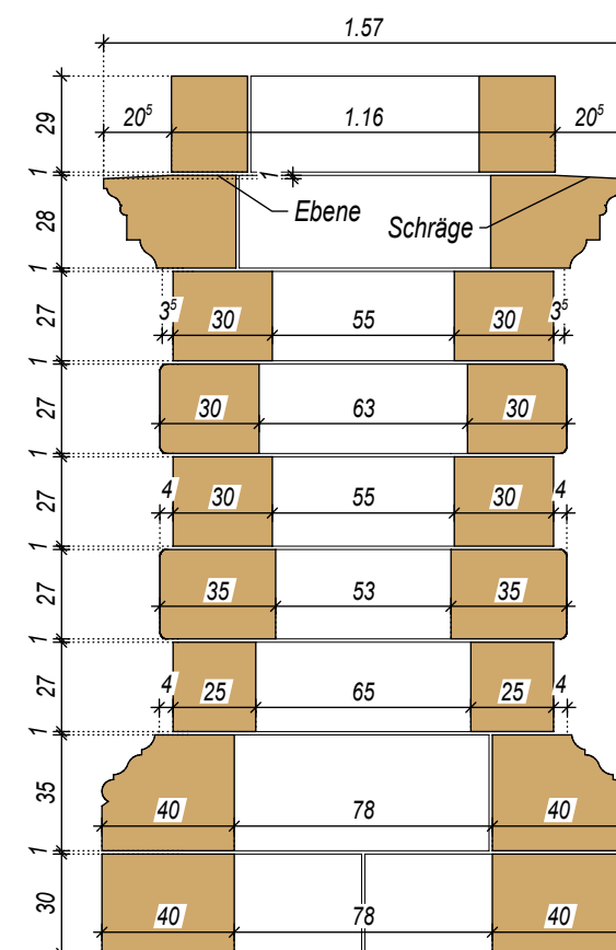
Schnitt SC2 - SC2 M = 1:25
