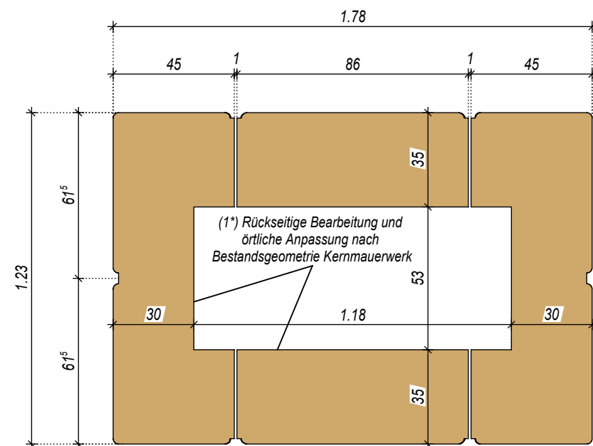
Schicht B1 - B1 M = 1:20 Bossen - Ausführung 1x
