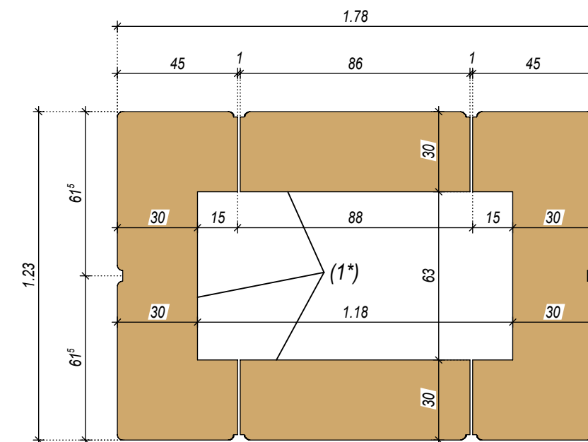
Schicht B2 - B2 M = 1:20 Bossen - Ausführung 1x
