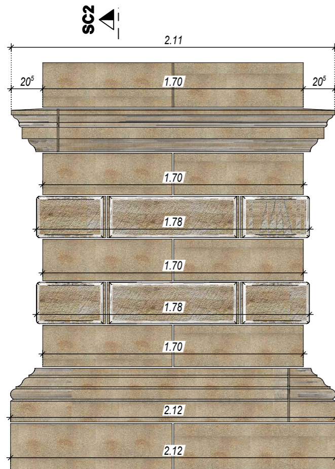
Ansicht Westen M = 1:25
