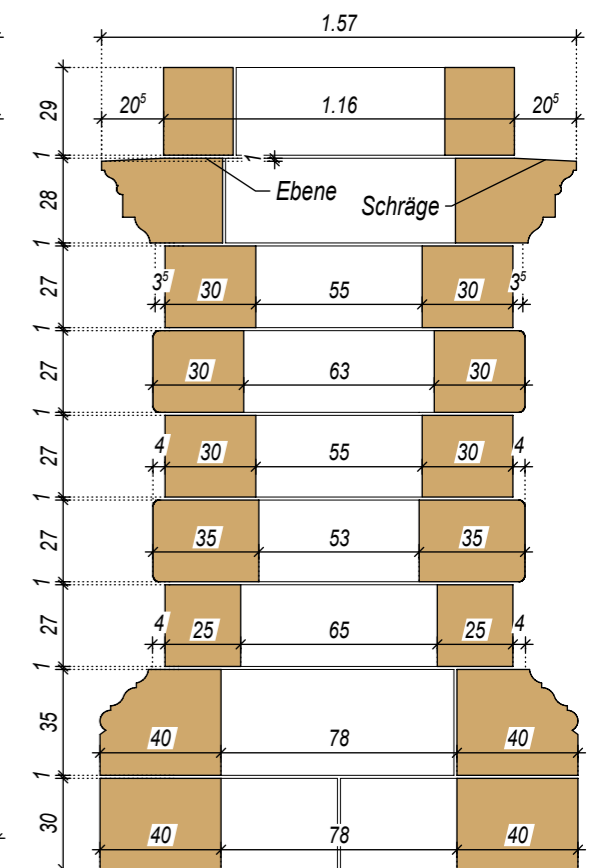
Schnitt SC2 - SC2 M = 1:25
