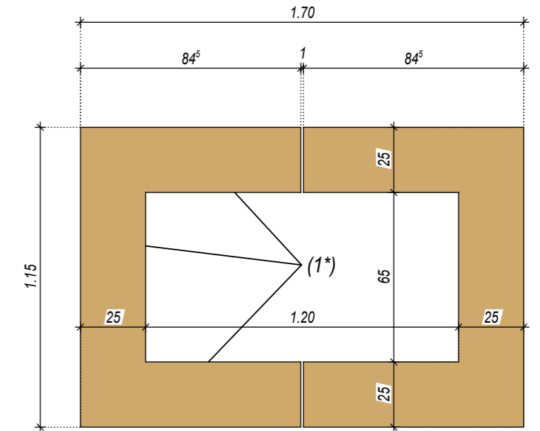
Schicht Q1 - Q1 M = 1:20 Quadermauerwerk - Ausführung 1x
