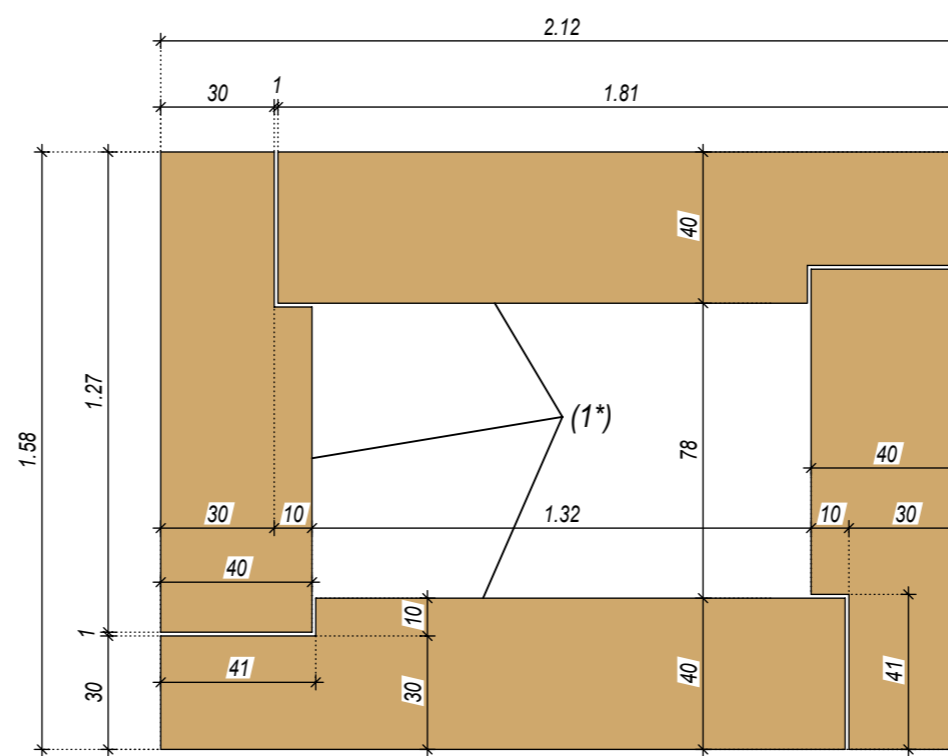
Schicht S2 - S2 M = 1:20 Sockelgesims - Ausführung 1x
