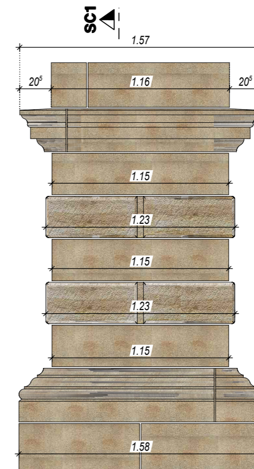
Ansicht Norden M = 1:25
