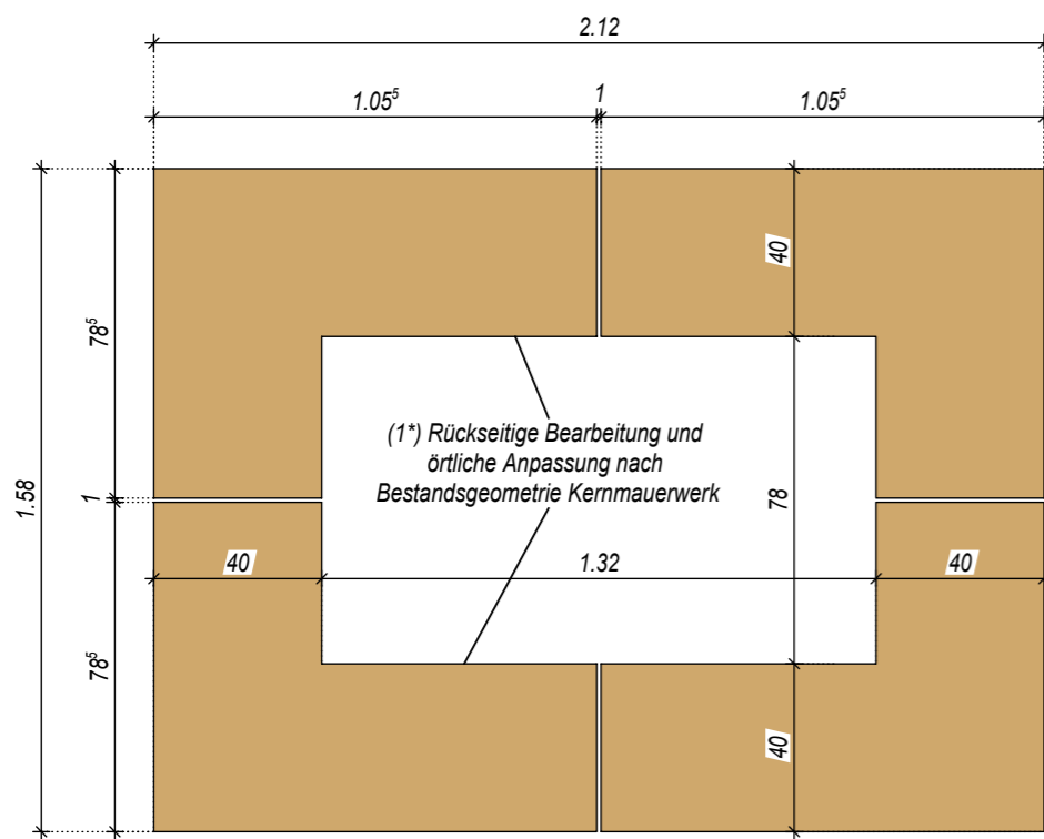
Schicht S1 - S1 M = 1:20 Quadermauerwerk Sockel - Ausführung 1x
