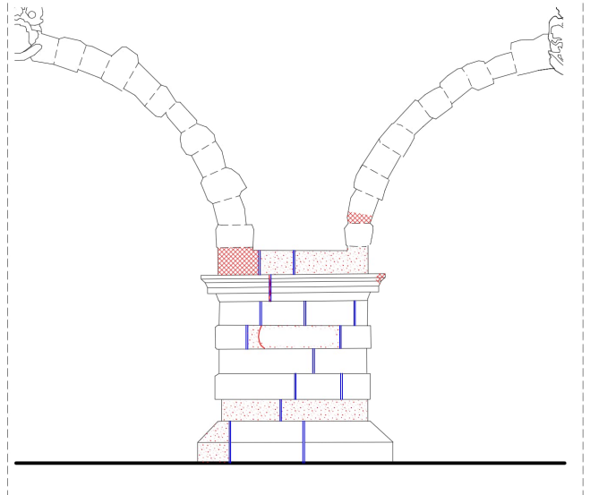
Ansicht West:
