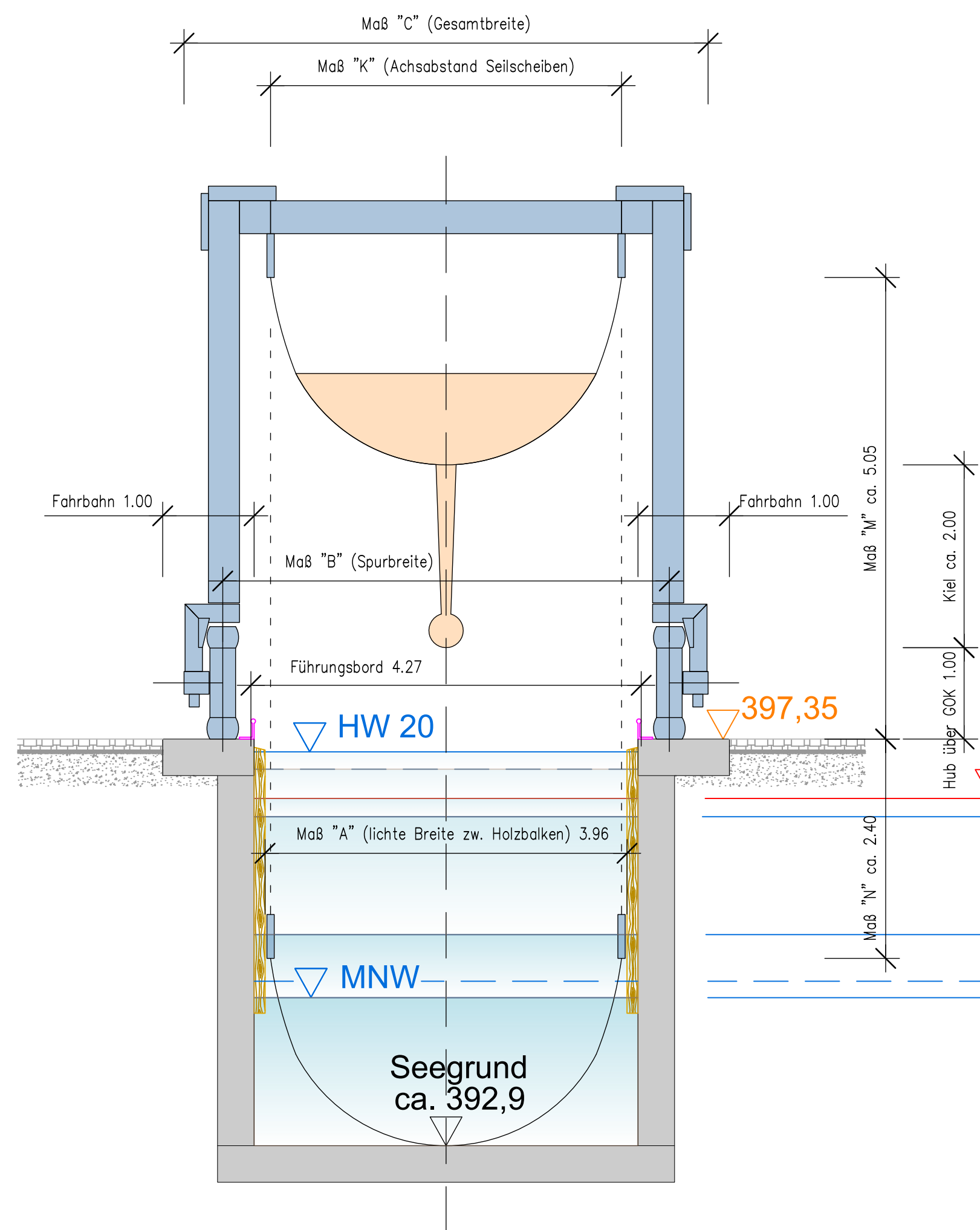
Querschnitt M 1:50
