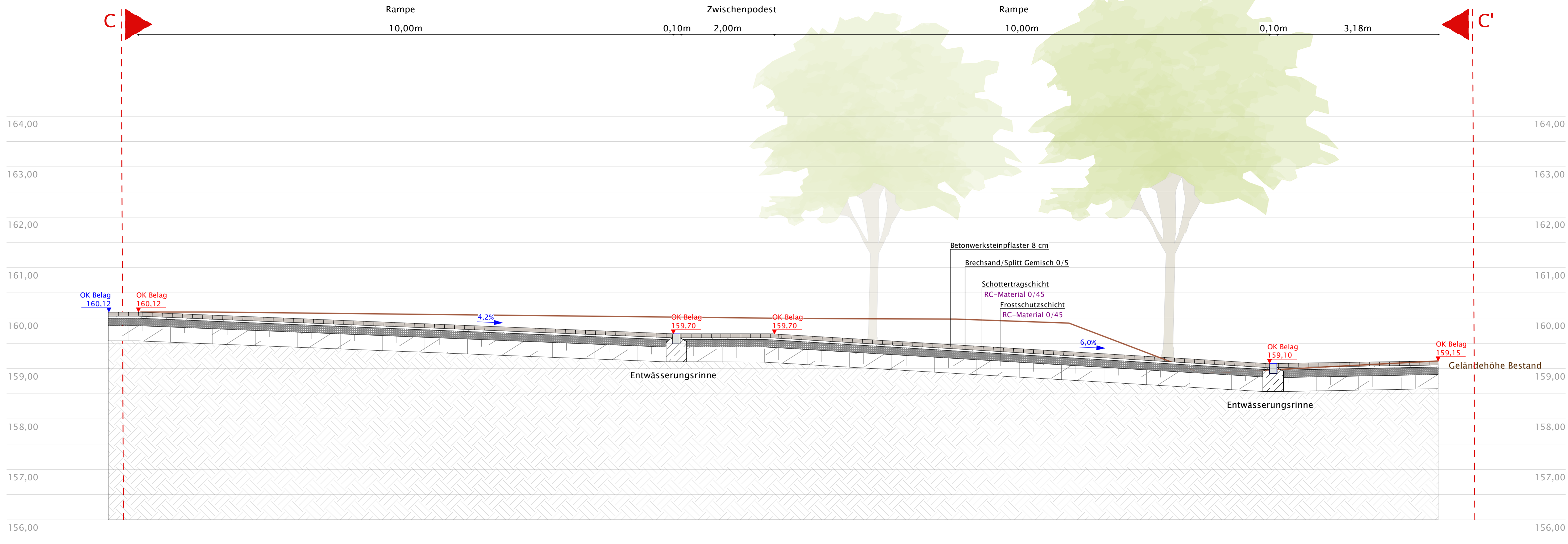
Schnitt CC' M 1:50
