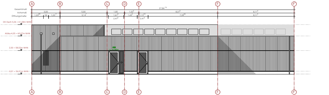
ANSICHT WEST
